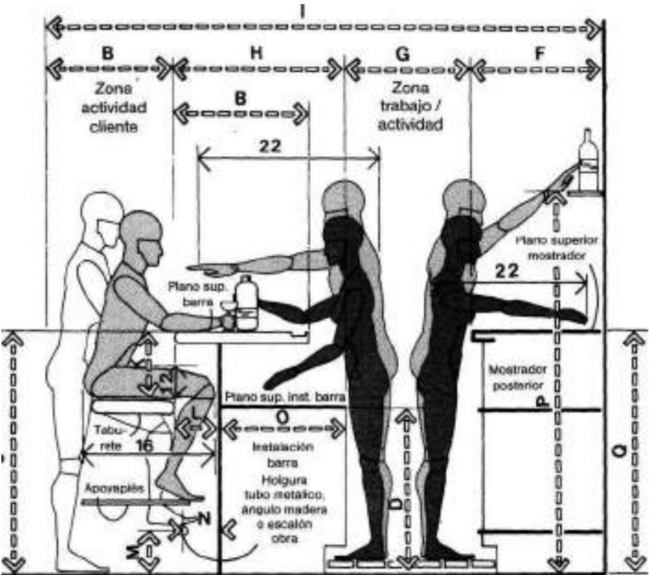
SECCIÓN DE BARRA
