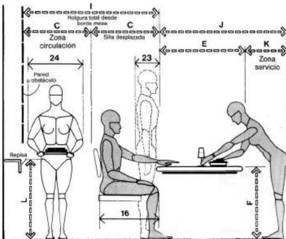
HOLGURA MÍNIMA PARA SILLA DESPLAZADA
