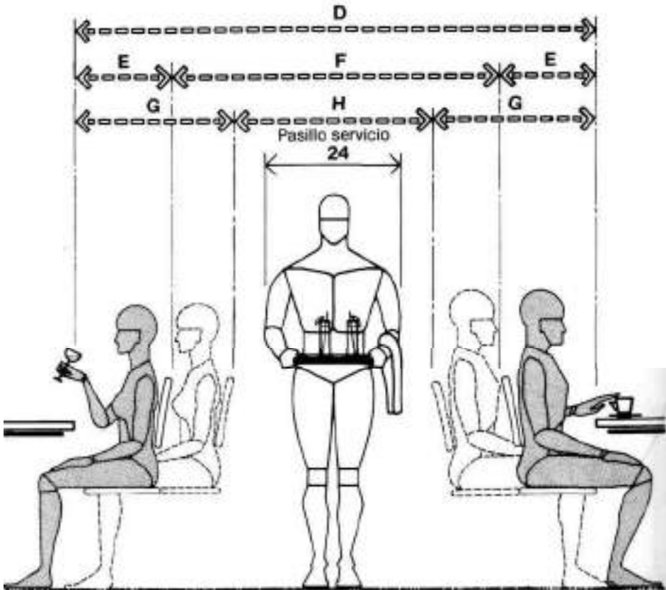
PASILLO DE SERVICIO/HOLGURA ENTRE SILLAS
