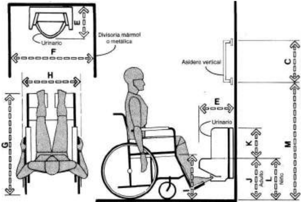
DISTRIB. DE URINARIO/USUARIO EN SILLA DE RUEDAS
