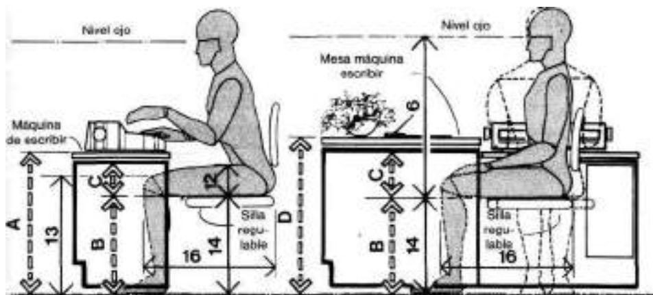
MODULO DE MECANOGRAFÍA Y MESA/HOMBRE
