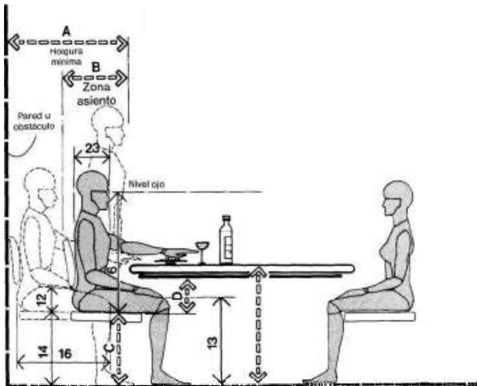
HOLGURA MÍNIMA PARA SILLA/SIN CIRCULACIÓN
