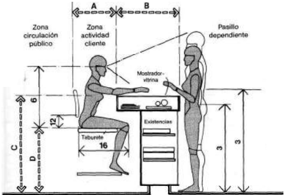
CLIENTE SENTADO/MOSTRADOR ALTO
