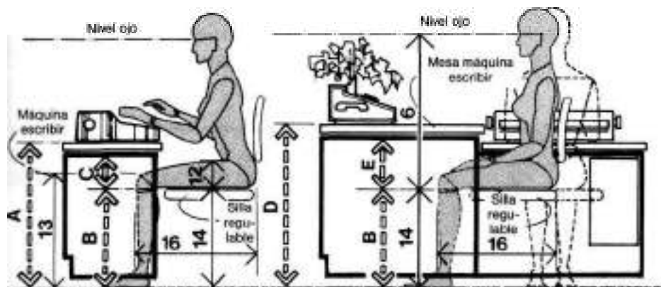
MODULO DE MECANOGRAFÍA/MUJER
