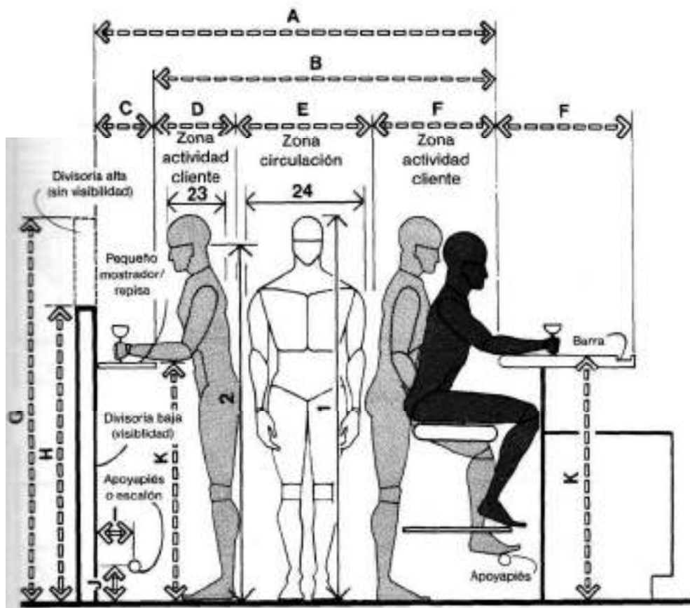
BARES/HOLGURA ZONA PÚBLICO
