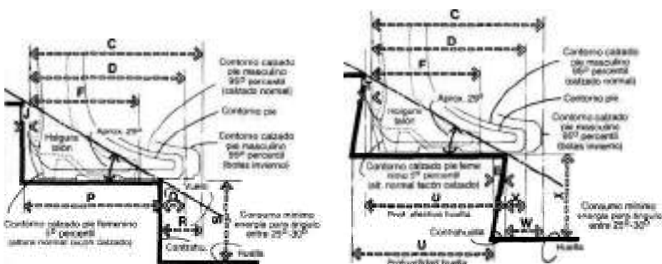
RELACIÓN HUELLA-CONTRAHUELLA/PROPORCIONES RECOMENDADAS (LEHMAN, 1962)
