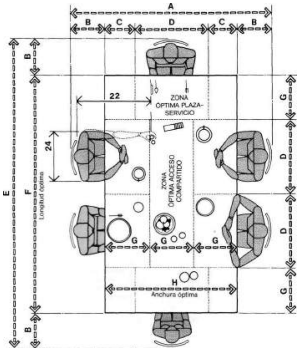
MESA RECTANGULAR/LONGITUD Y ANCHURA MÍNIMA/SEIS PERSONAS
