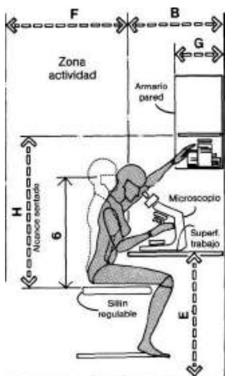
ZONA DE LABORATORIO/CONSIDERACIONES FEMENINAS
