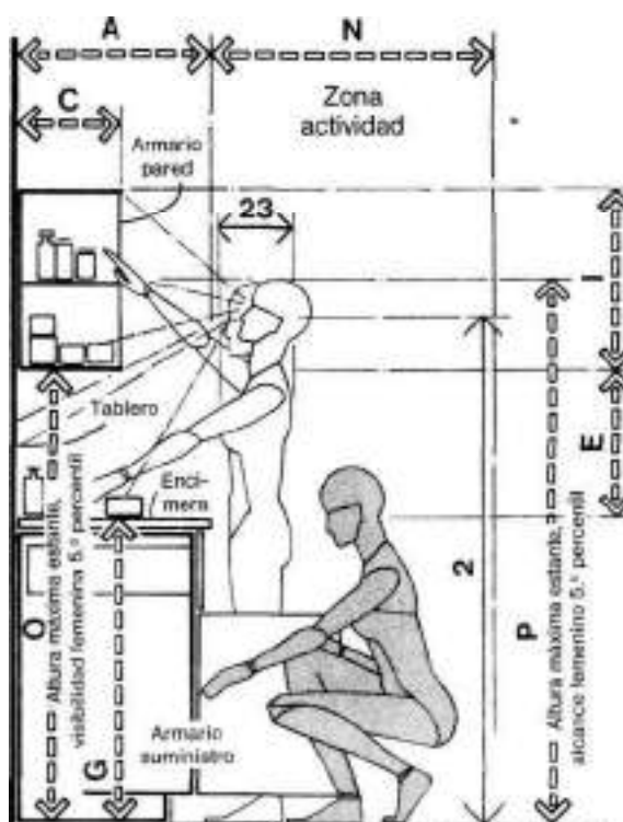
ARMARIO INSTR. Y SUMINISTRO/CONSIDERACIONES FEMENINAS
