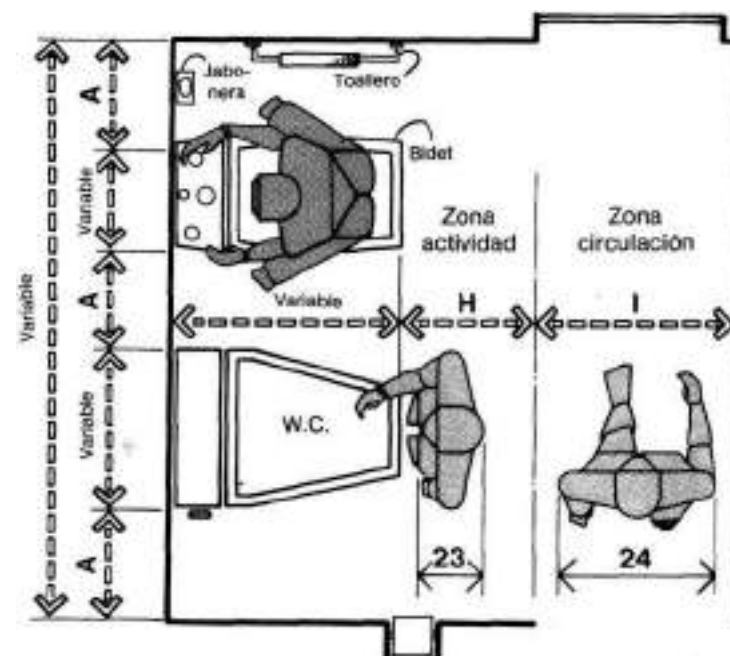
BIDET Y TOALLERO
