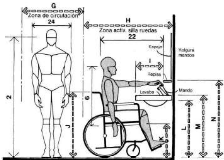
LAVABO/USUARIO EN SILLA DE RUEDAS
