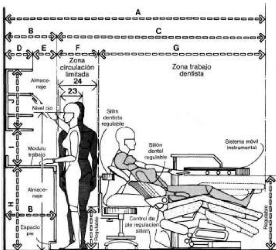
ESPACIO DE TRATAMIENTO/CONSIDERACIONES VERTICALES
