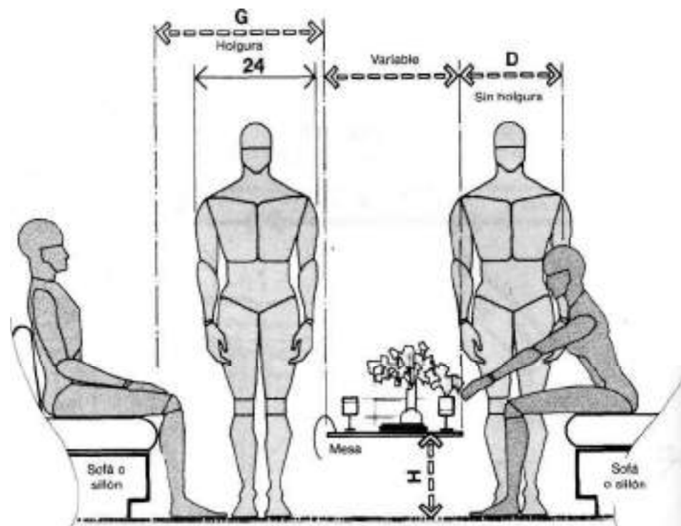
ASIENTOS ESTAR/RELACION HOLGURAS
