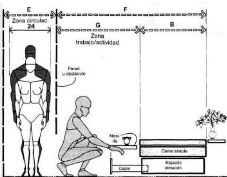
CAMA SIMPLE/HOLGURAS Y DIMENSIONES
