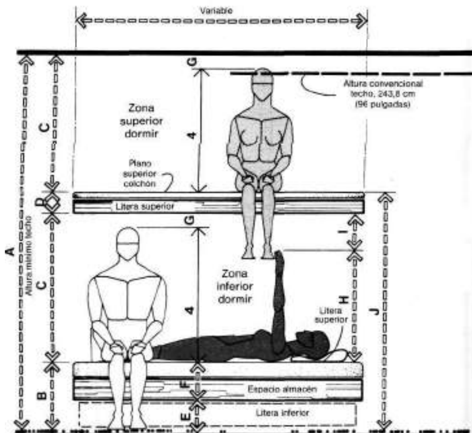
LITERAS PARA ADULTOS / ALZADO FRONTAL
