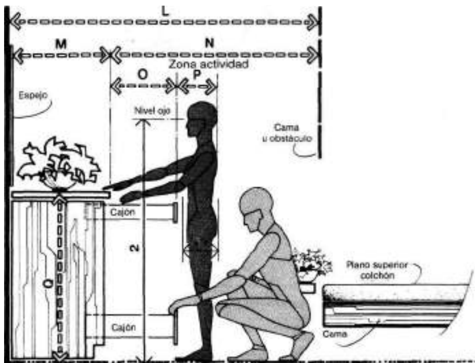
HOLGURA CÓMODA / CAMA
