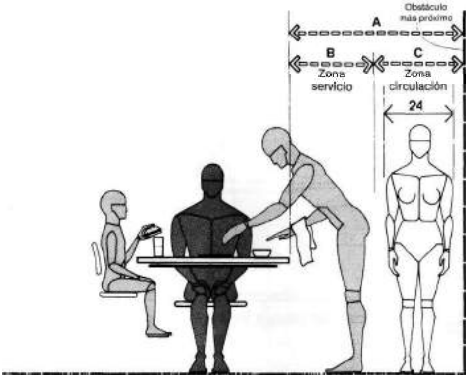
MESAS/HOLGURA PARA EL CAMARERO Y LA CIRCULACIÓN
