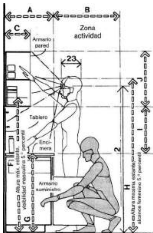
ARMARIO DE INSTRUMENTOS Y SUMINISTRO/CONSIDERACIONES MASCULINAS
