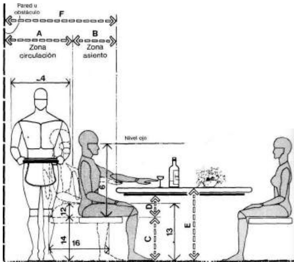
HOLGURA MÍNIMA DETRAS DE LA SILLA
