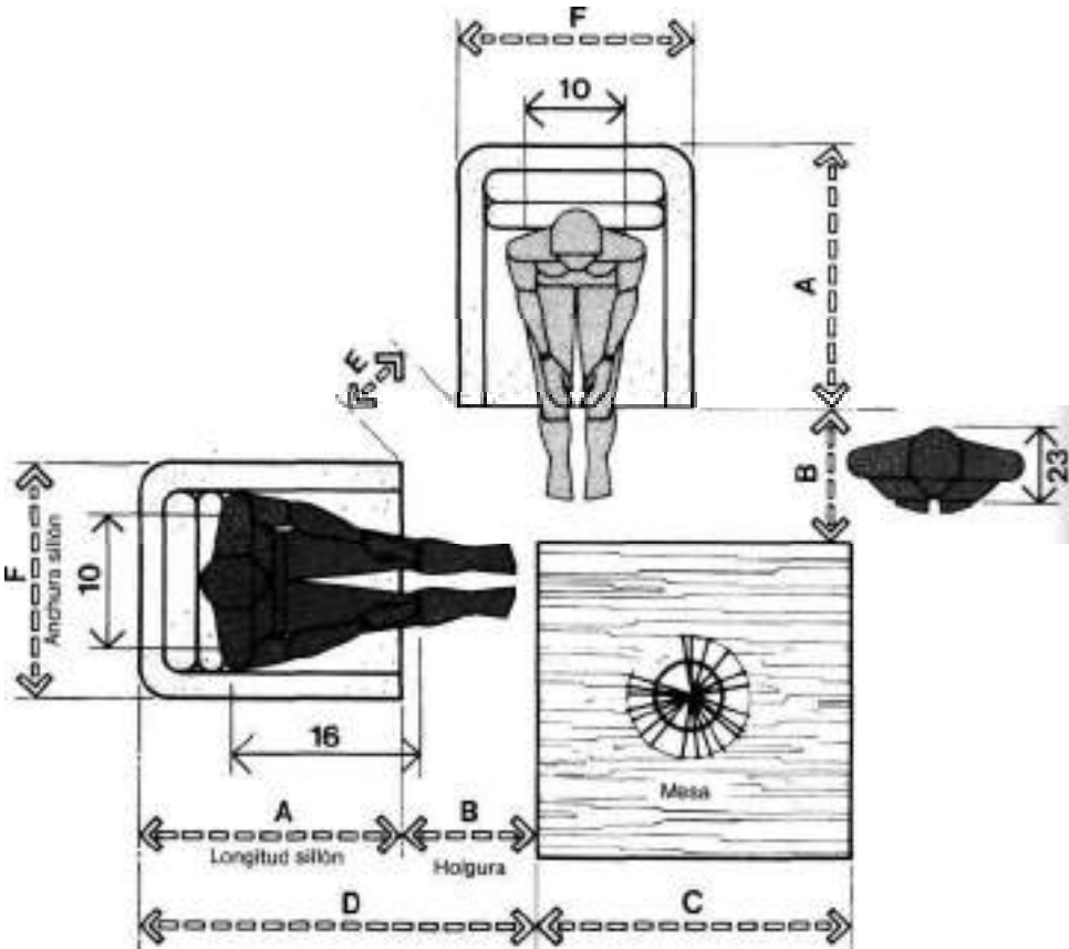
MÓDULO DE ESPERA EN RECEPCIÓN
