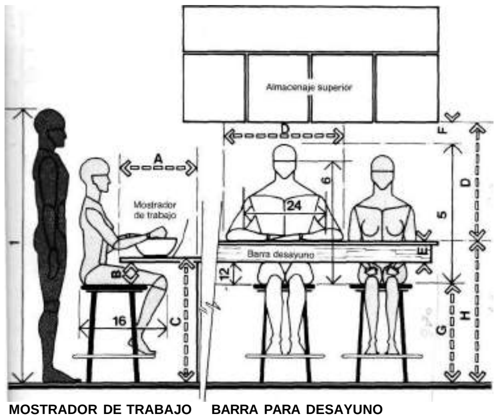
MOSTRADOR DE TRABAJO BARRA PARA DESAYUNO
