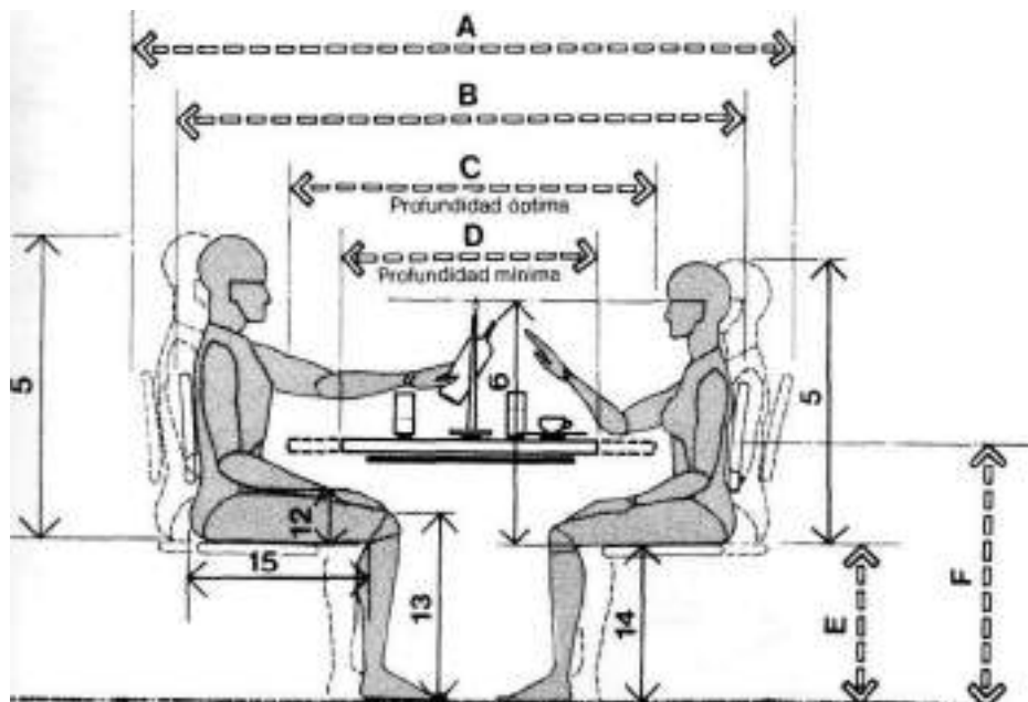
MESAS / PROFUNDIDAD MÍNIMA Y ÓPTIMA / HOLGURAS VERTICALES
