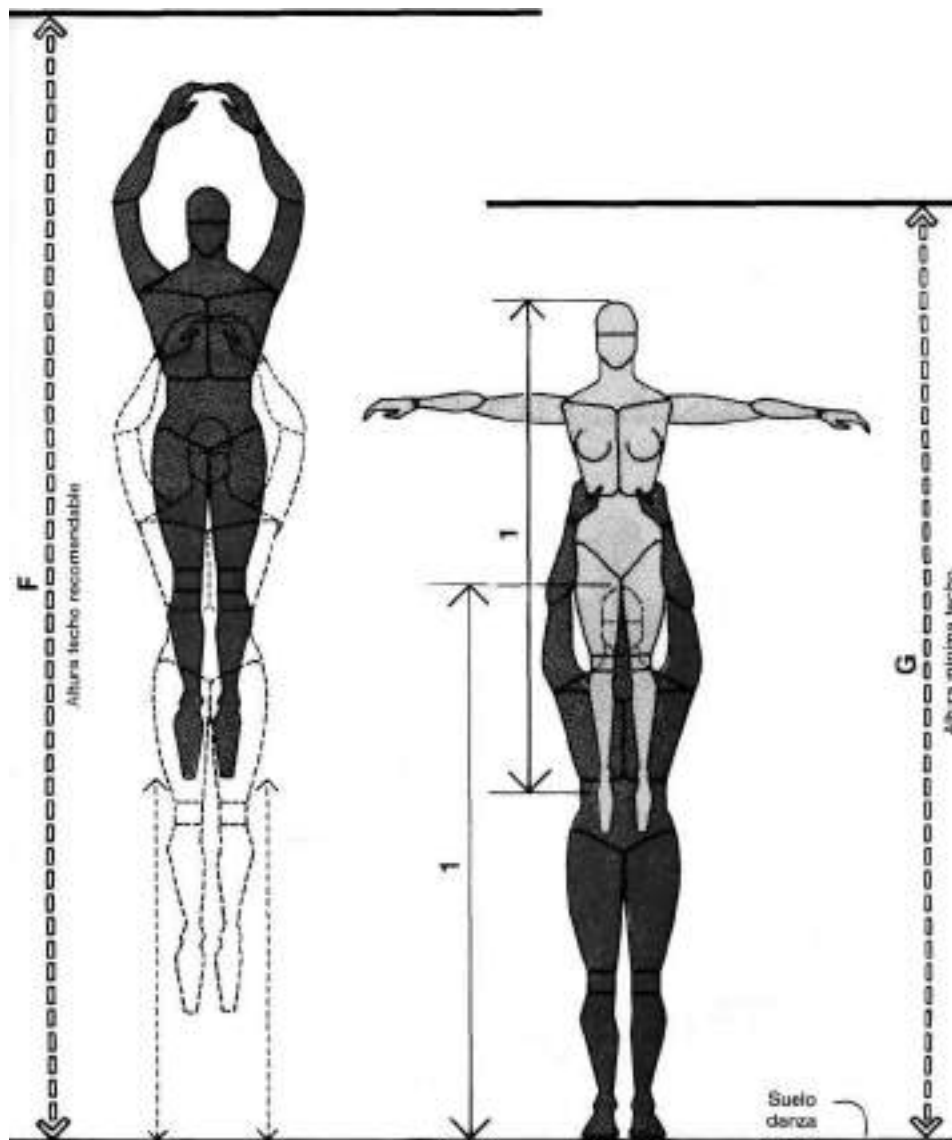
ESPA. PARA DANZA Y PRÁCT. DE EJERCICIOS/ REQUISITOS DE ALTURA DE TECHO
