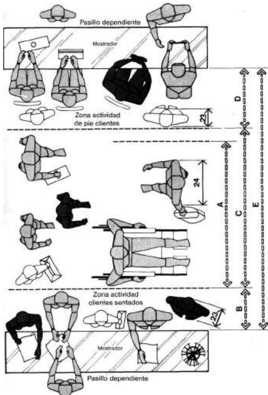
ANCHURAS DE PASILLOS PÚBLICOS PRINCIPALES
