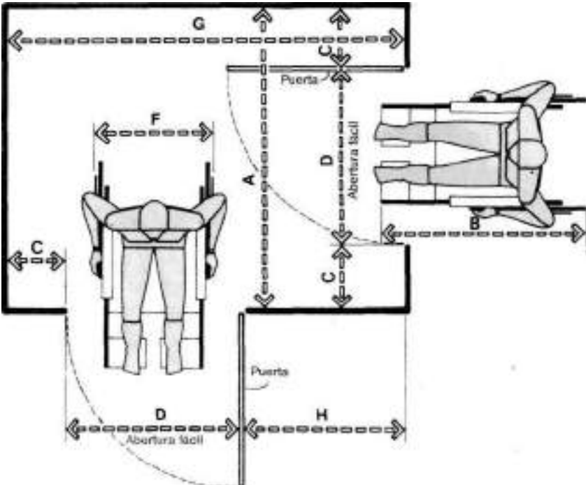
CiRCULACiÓN EN SILLA RUEDAS/PUERTAS EN PARAMENTOS PERP,
