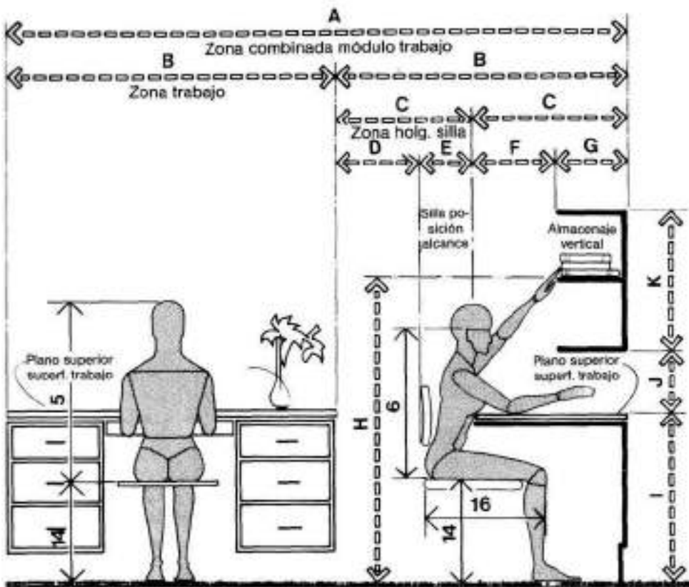
MODULO BÁSICO DE TRABAJO CON ALMACENAJE VERTICAL
