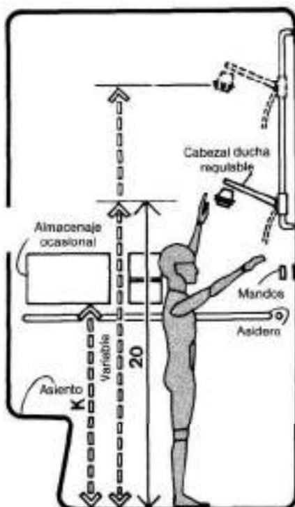
CONSIDERACIONES ANTROPOMÉTRICAS DUCHA/BAÑO
