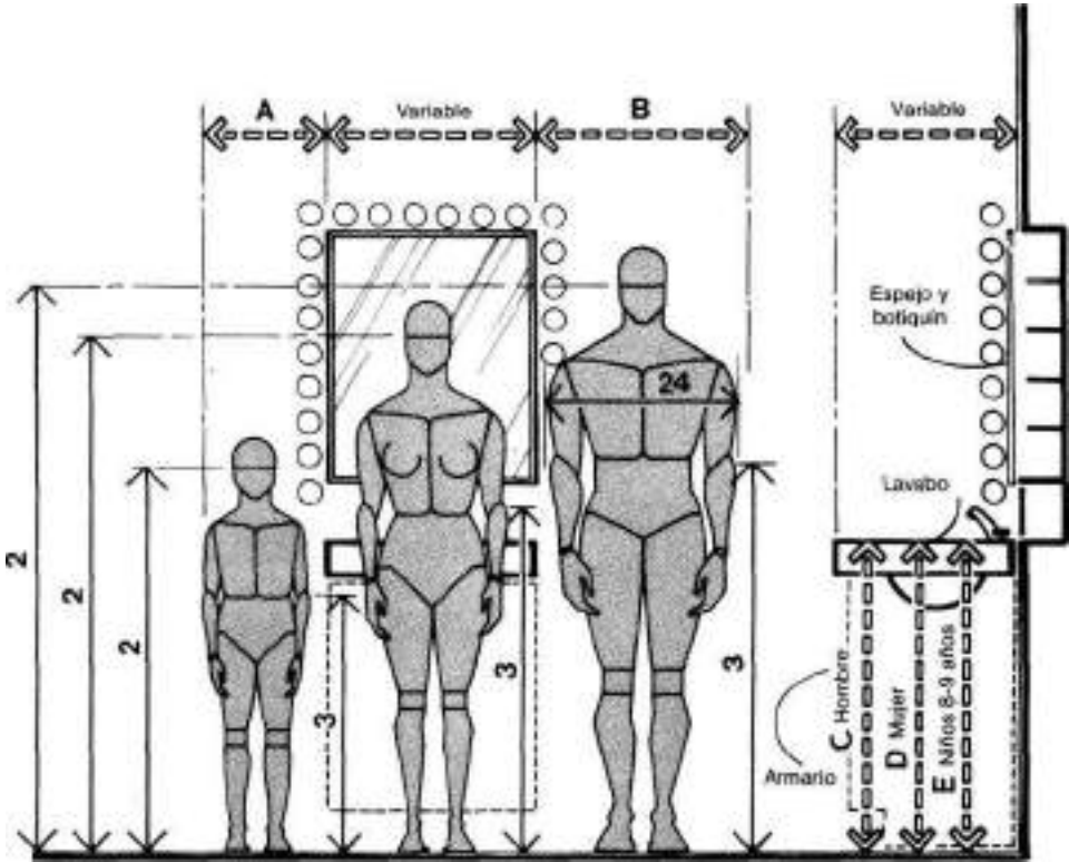
LAVABO/CONSIDERACIONES ANTROPOMÉTRICAS GENERALES
