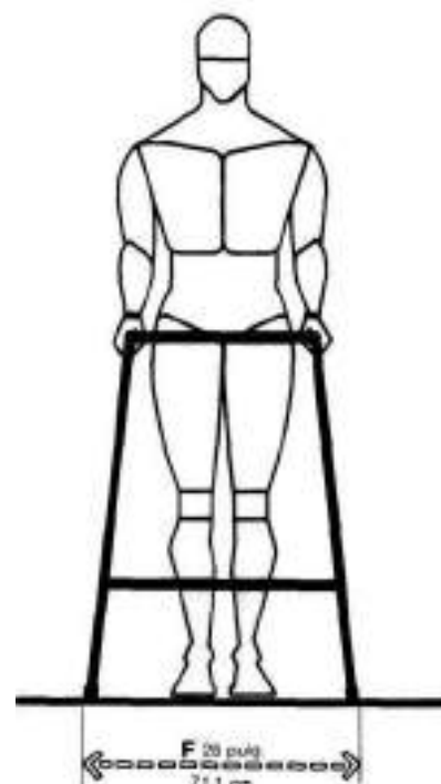
Fig. 3-6. Andador. La holgura que requiere un usuario que se ayuda con andador se define fácilmente a causa de la propia naturaleza del dispositivo y método de utilización. La vista frontal del usuario indica un mínimo para (F) de 71,1 cm (28 pulgadas).
