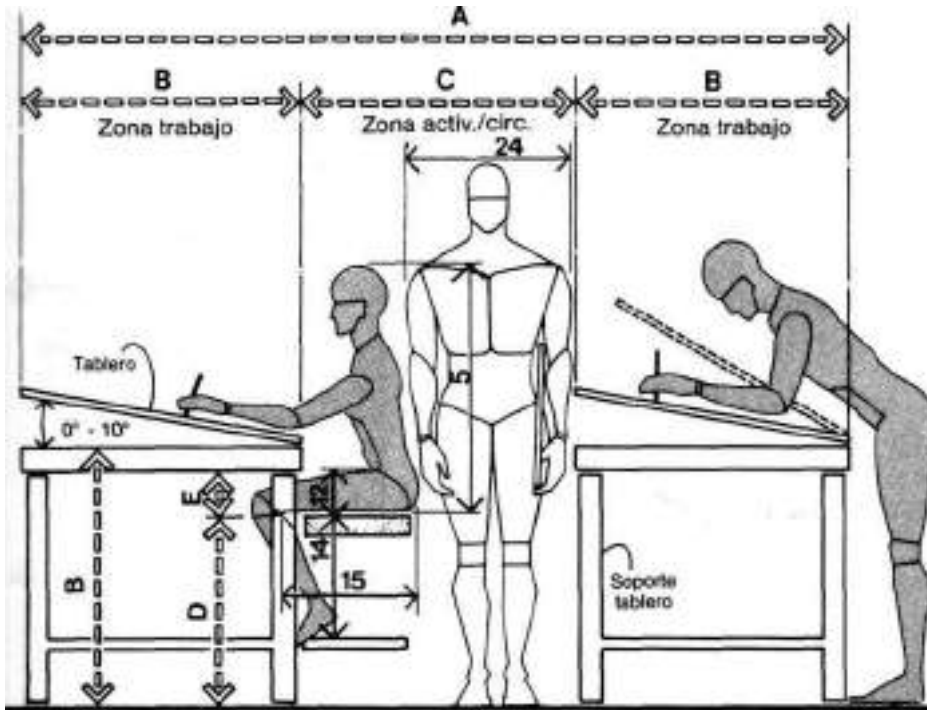
MESAS DE DIBUJO/HOLGURAS
