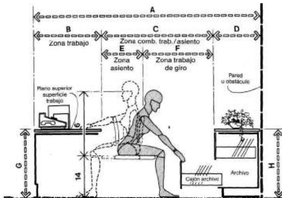
MODULO DE TRABAJO CON ARCHIVO POSTERIOR
