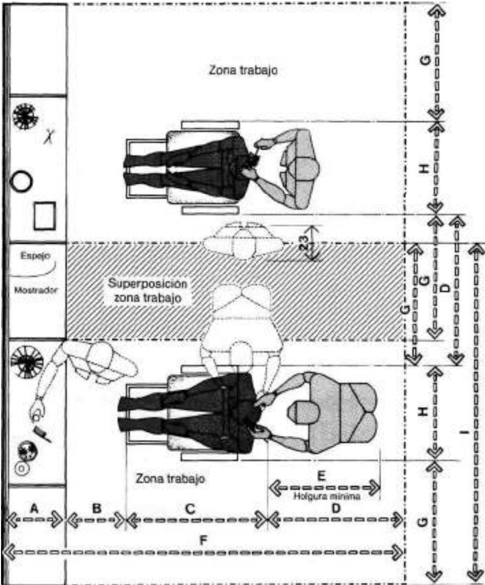
MÓDULOS DE TRABAJO EN PELUQUERÍA
