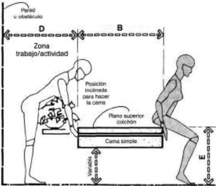
CAMA SIMPLE/HOLGURAS Y DIMENSIONES
