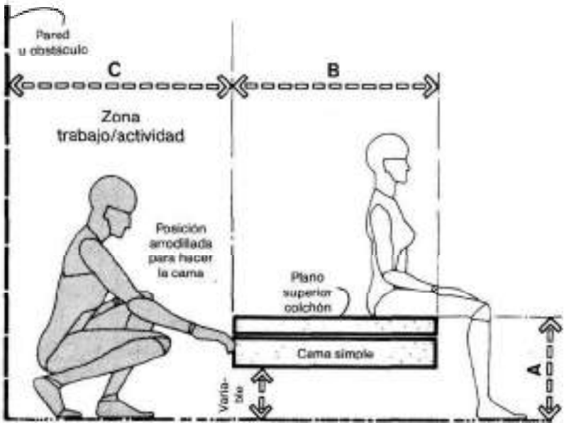
CAMA SIMPLE/HOLGURAS Y DIMENSIONES
