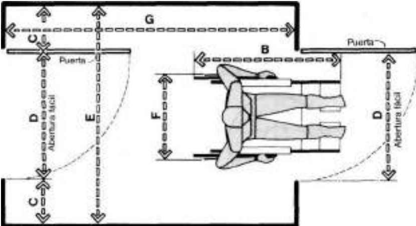
CIRCULACIÓN EN SILLA DE RUEDAS/PUERTAS ALINEADAS
