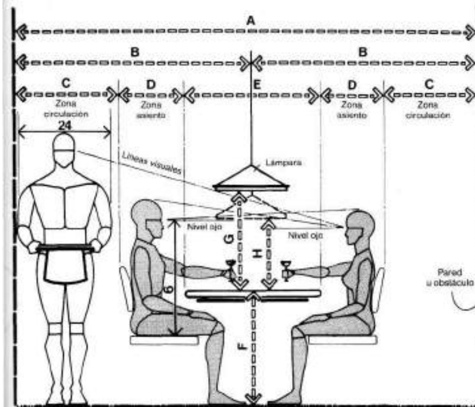
ANCHURA MÍNIMA DE LA ZONA PARA COMER
