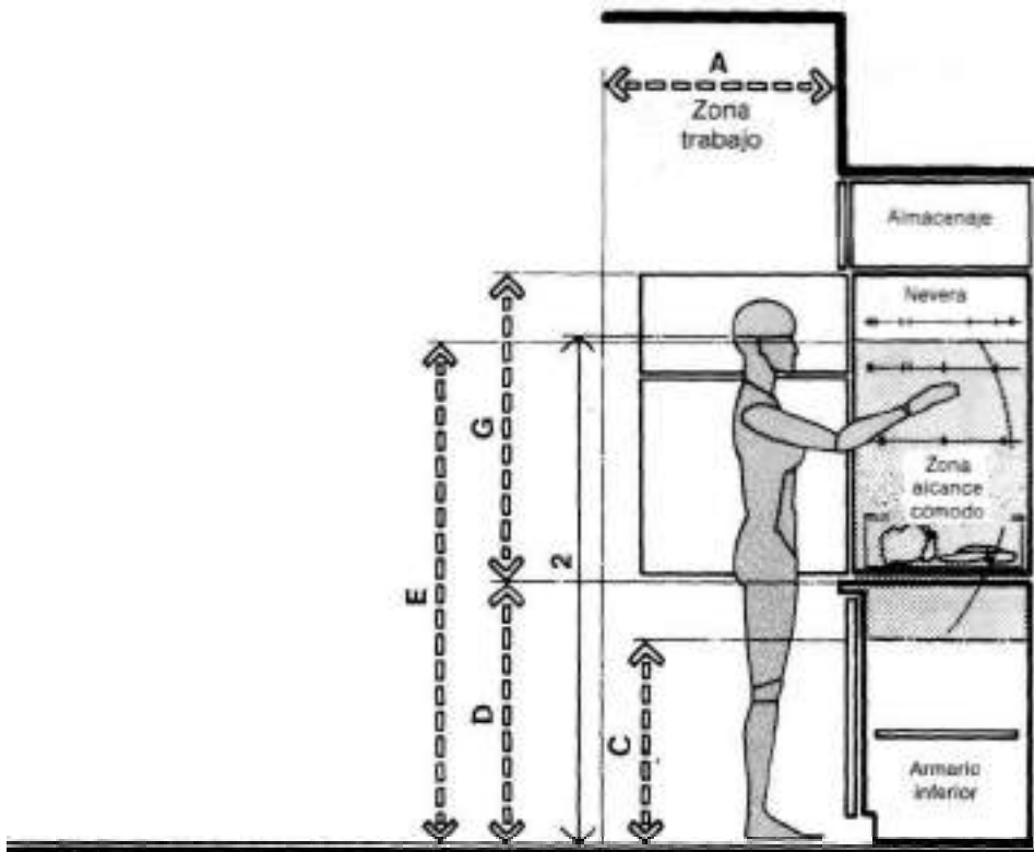
NEVERA/PROPUESTA DE EMPLAZAMIENTO
