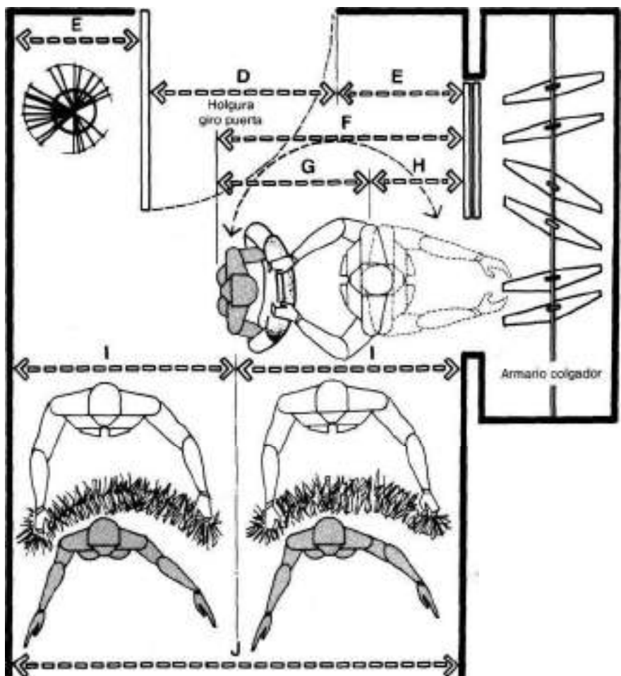
VESTÍBULO/HOLGURAS PARA DESPOJARSE DE ABRIGOS
