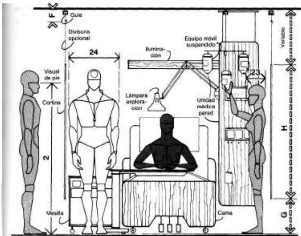
CUBÍCULO CON CAMA DE PACIENTE Y CORTINAS DIVISORIAS
