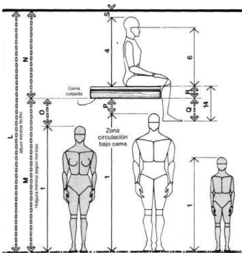
CAMAS COLGADAS / ALZADO LATERAL
