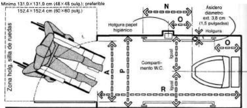
COMPAT. DEL INODORO/ACCESO CON TRANSF. FRONTAL
