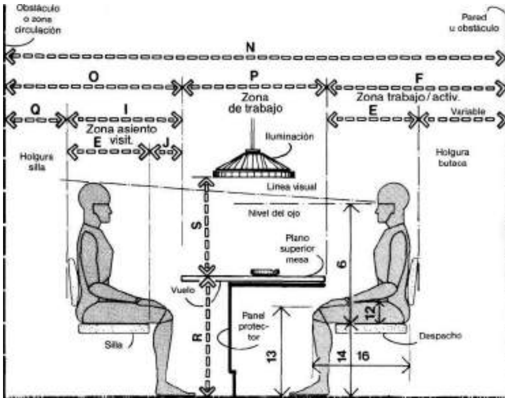
MESA DE DESPACHO/HOLGURAS BÁSICAS
