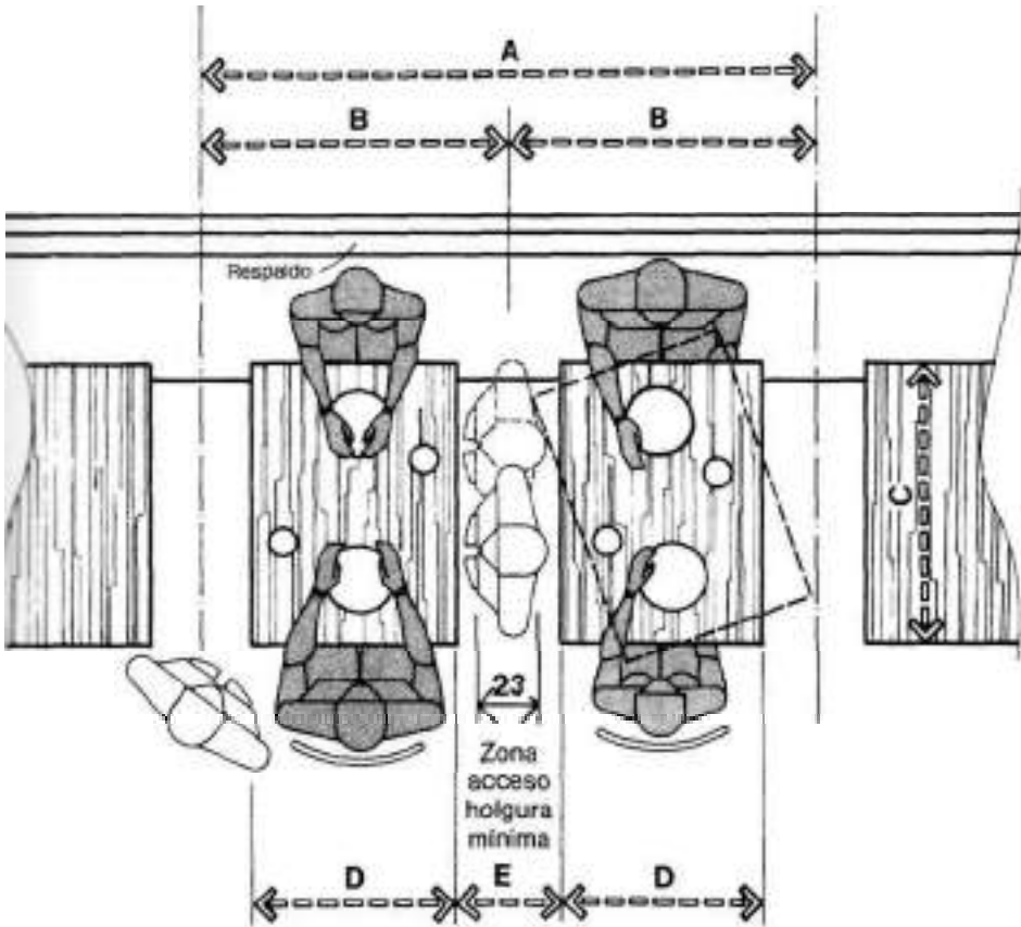
BANCO CORRIDO/HOLGURAS MÍNIMAS
