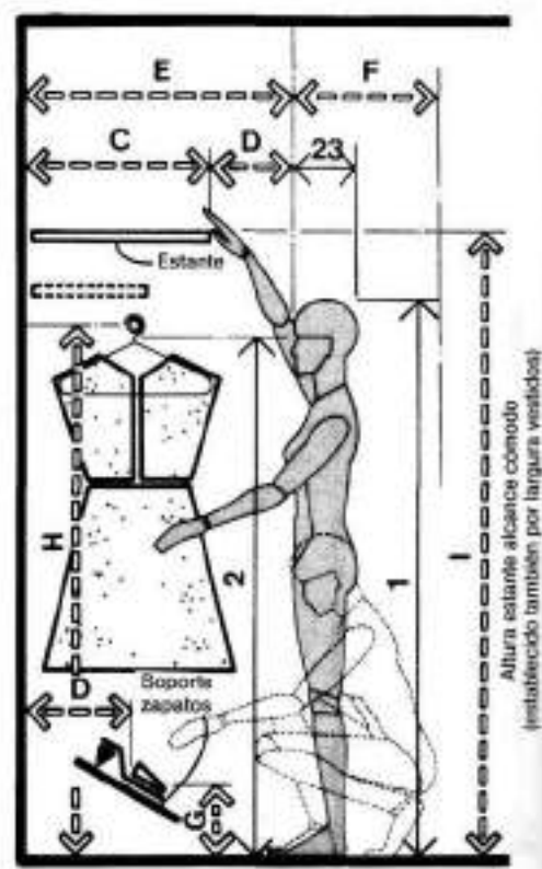
CLOSET Y ALMACENAJE/ MUJER
