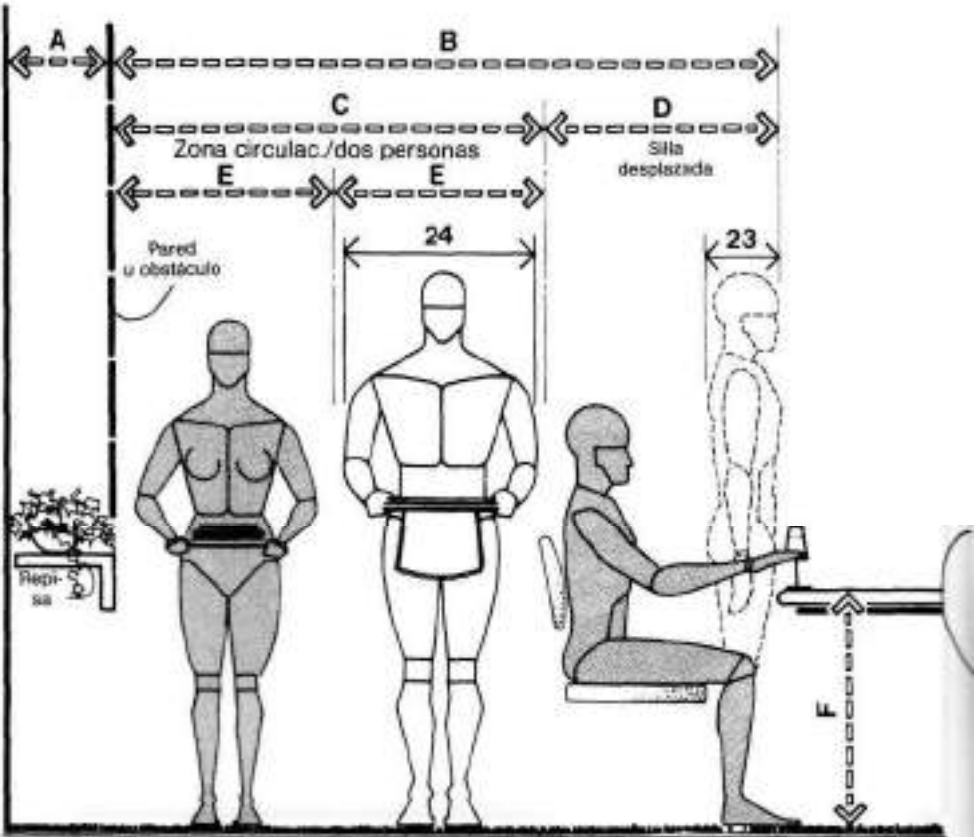
HOLGURA MÍNIMA DETRÁS DE DOS SILLAS DESPLAZADAS
