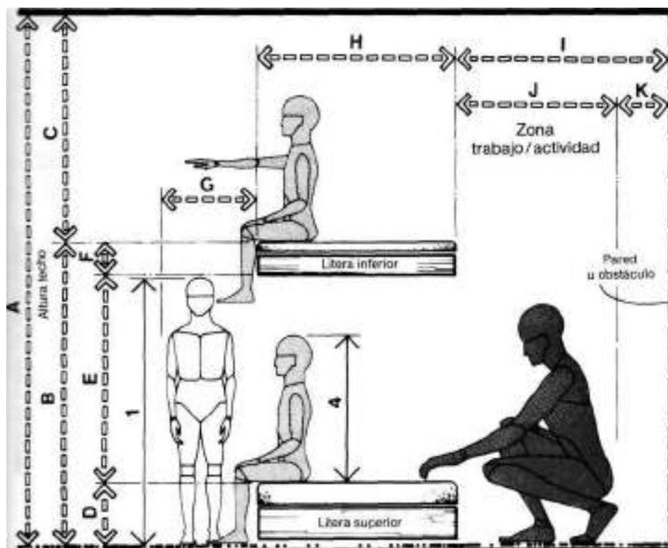
LITERAS PARA NIÑOS/ALZADO LATERAL
