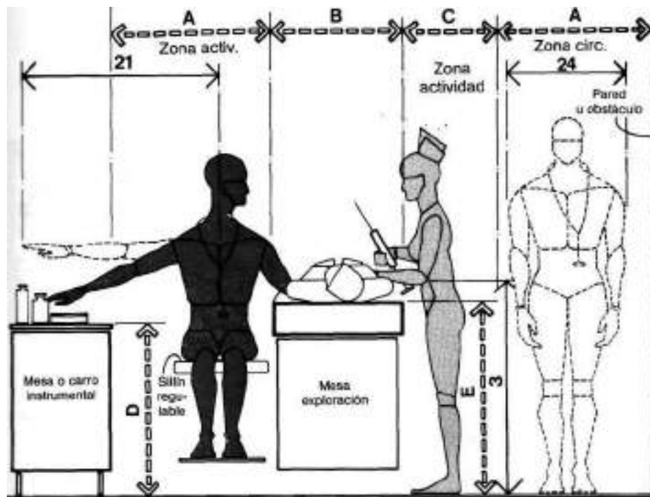
ZONA DE EXPLORACIÓN/ALCANCE Y HOLGURA
