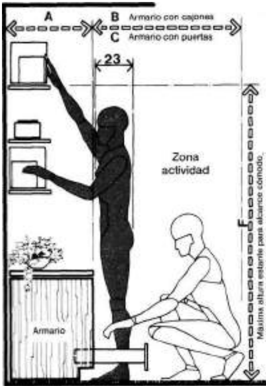
MUEBLE PARED/ACCESO HOMBRE
