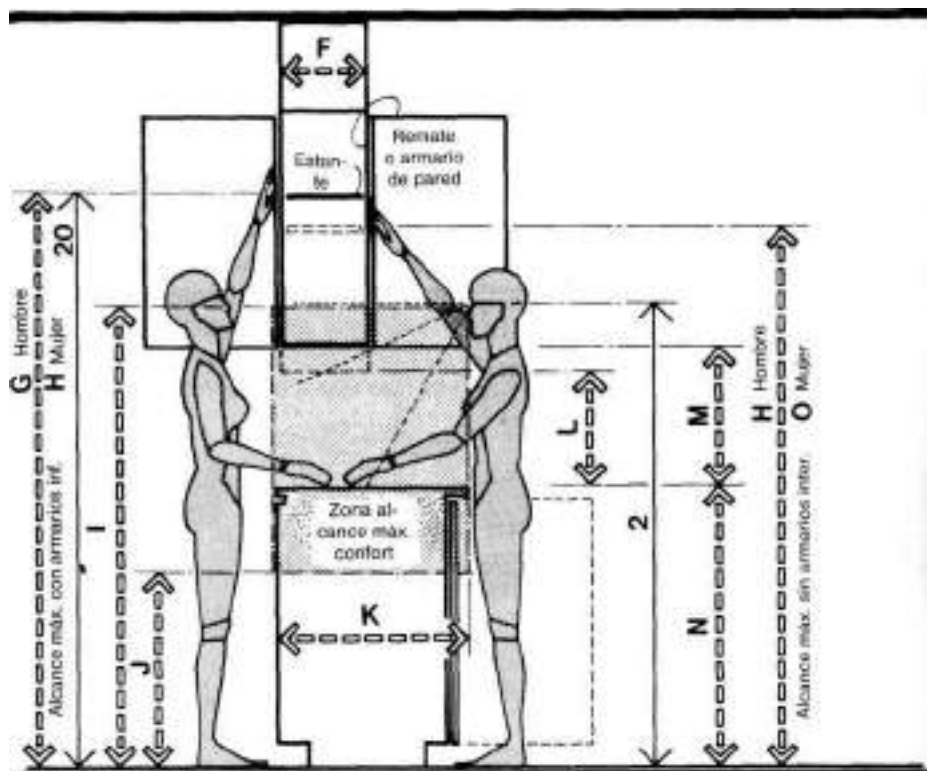
ALCANCE COMPARATIVO EN ARMARIOS DE COCINA
