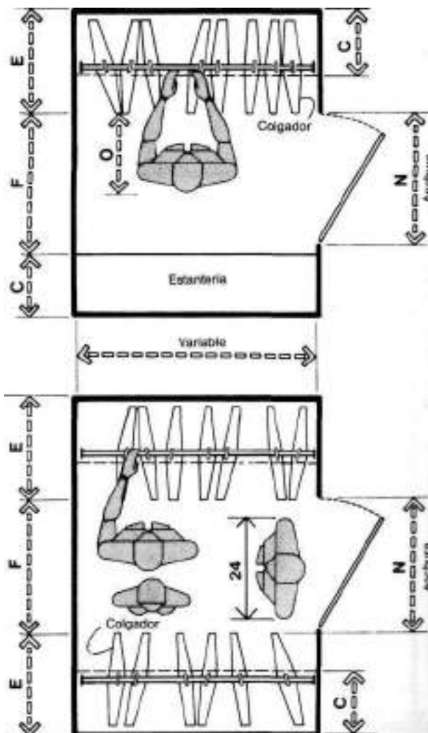
CLOSET Y ALMACENAJE CON ACCESO INTERIOR
