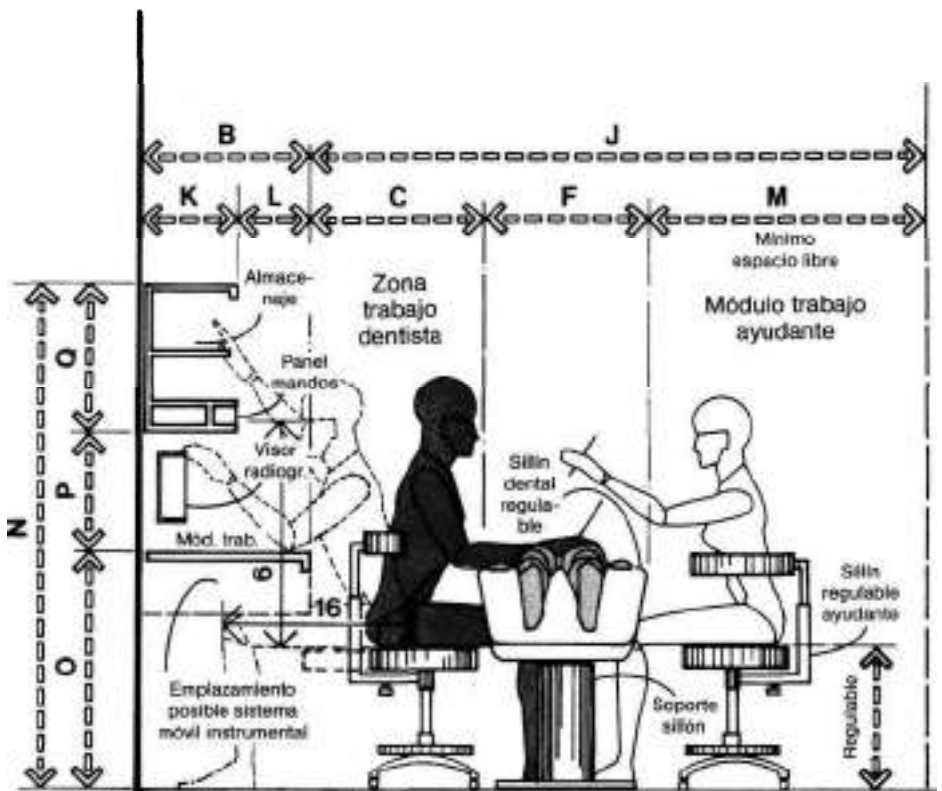
ESPACIO DE TRATAMIENTO/CONSIDERACIONES VERTICALES
