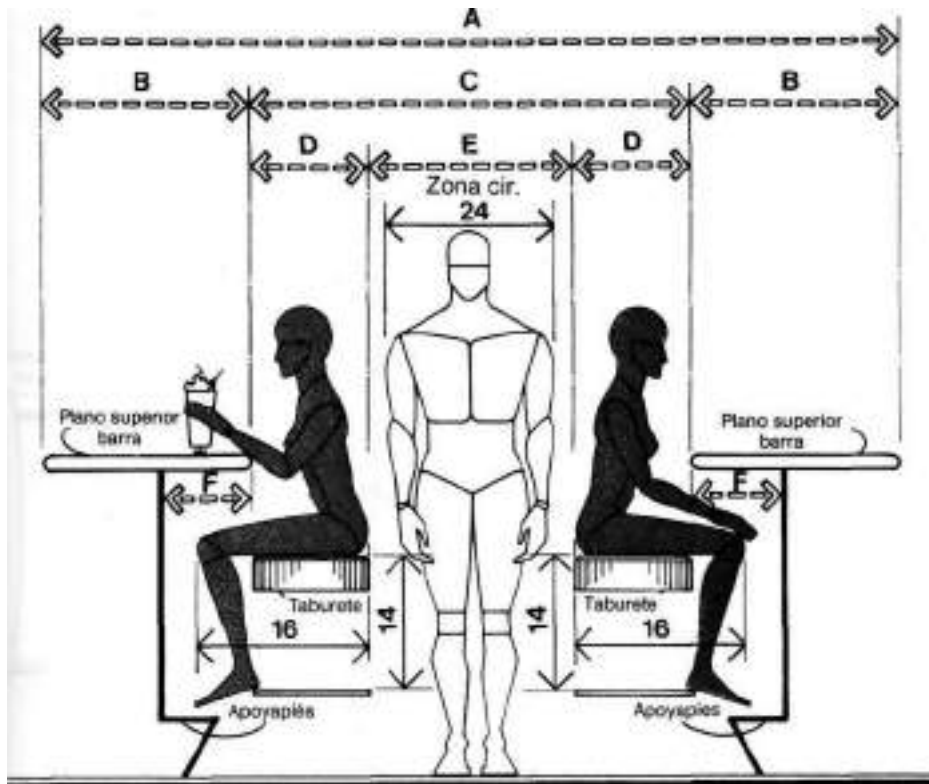
BARRA PARA COMER/HOLGURA ENTRE TABURETES
