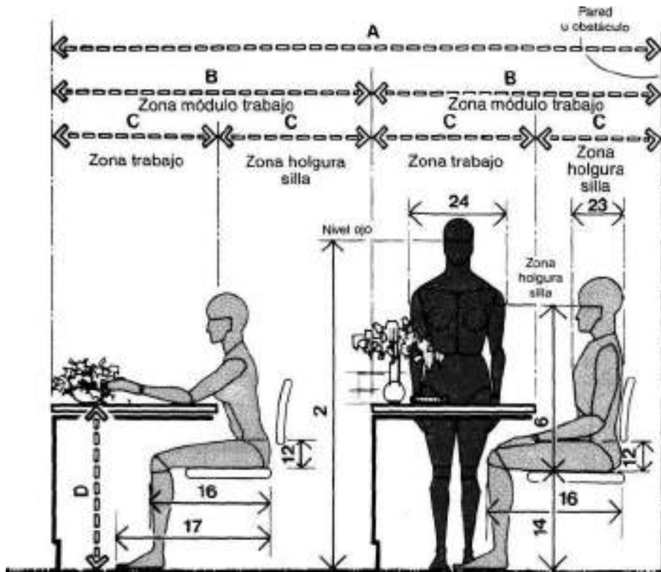
MÓDULOS DE TRABAJO ADYACENTES/DISTRIBUCIÓN EN HILERA
