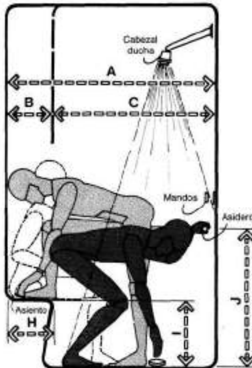
HOLGURAS MÍNIMAS PARA DUCHAS
