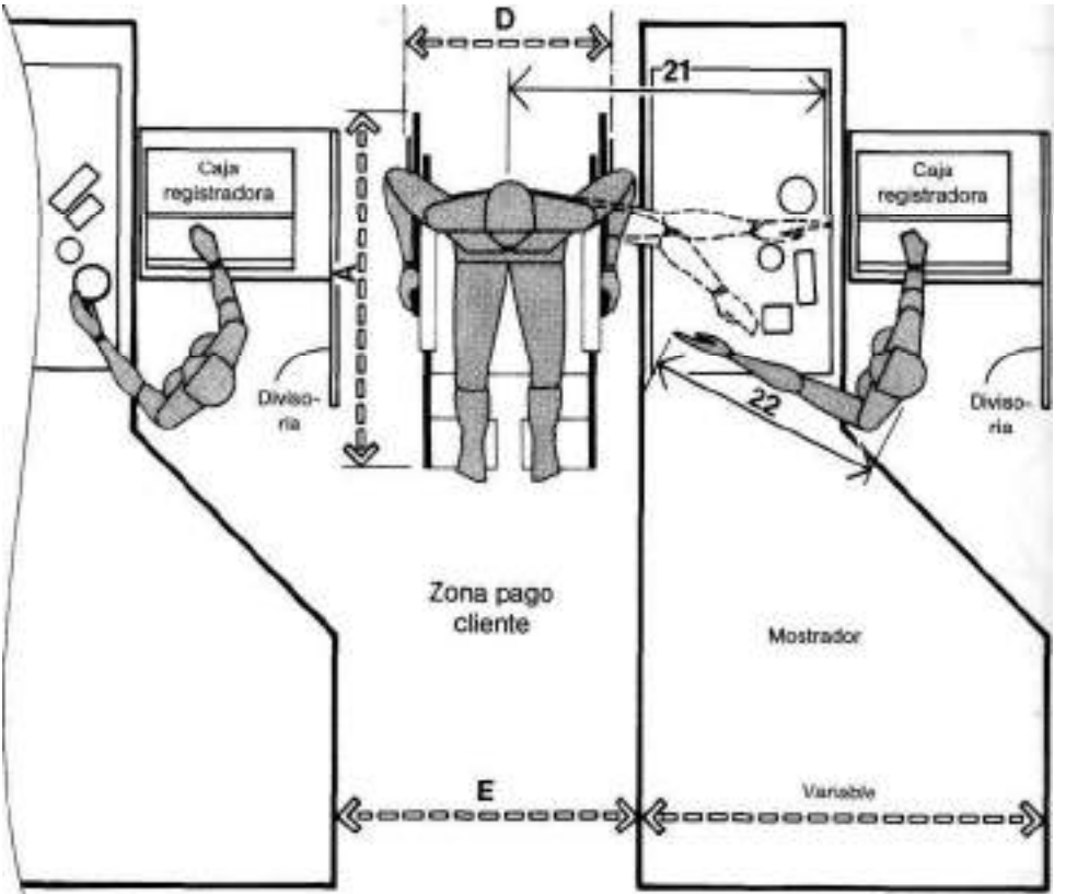
ZONA DE PAGO/HOLGURA PARA SILLA DE RUEDAS
