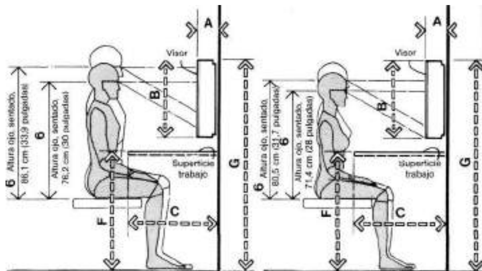
ALTURA OJO/OBSERVADORES SENTADOS, AMBOS SEXOS, ALTOS Y BAJOS
