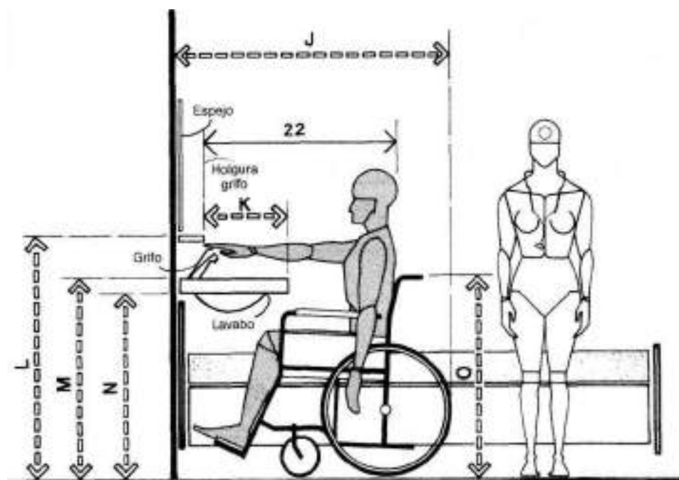
LAVABO DEL DORMITORIO
