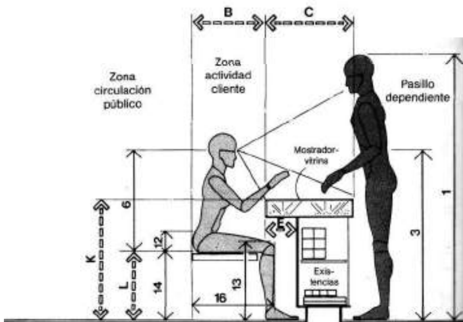
CLIENTE SENTADO/MOSTRADOR BAJO
