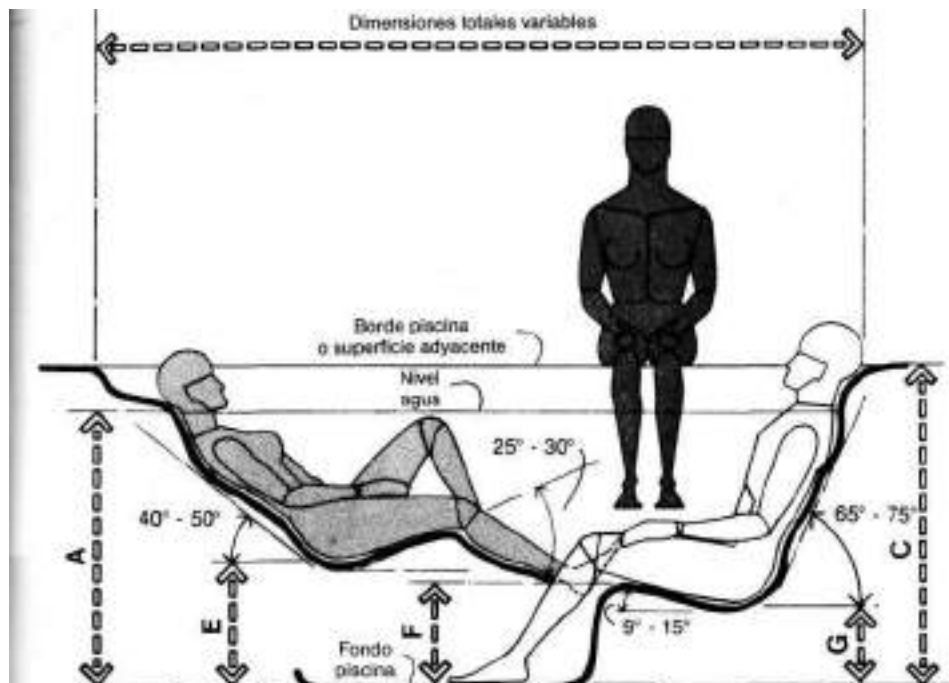
PISCINA PARA HIDROTERAPIA DE DIMENSIONES ANTROPOMÉTRICAS
