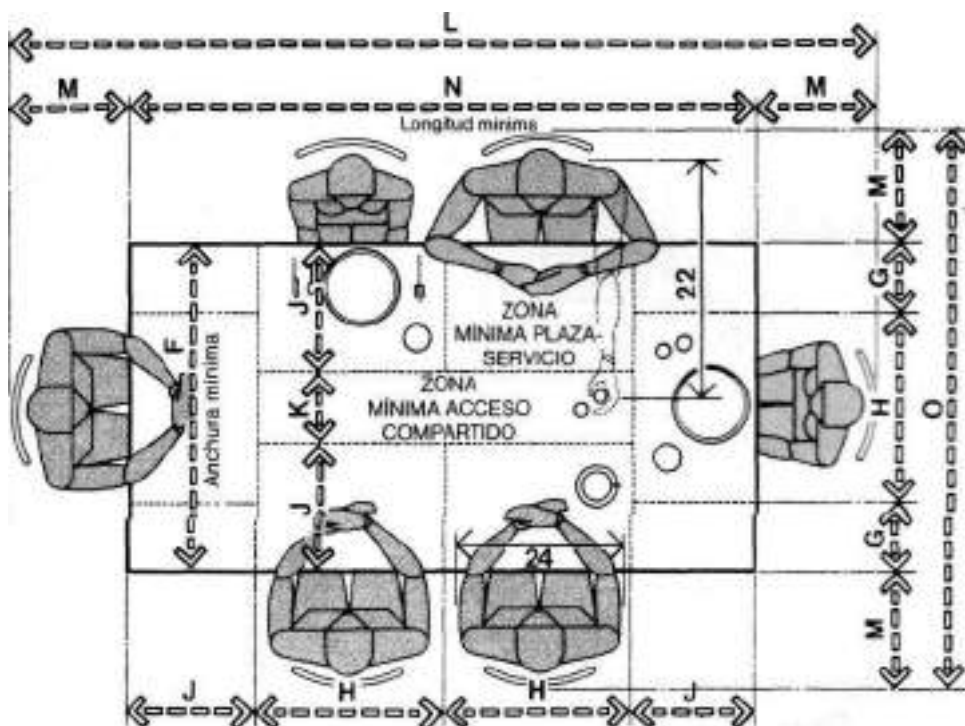
MESA RECTANGULAR / LONGITUD Y ANCHURA MÍNIMA/SEIS PERSONAS
