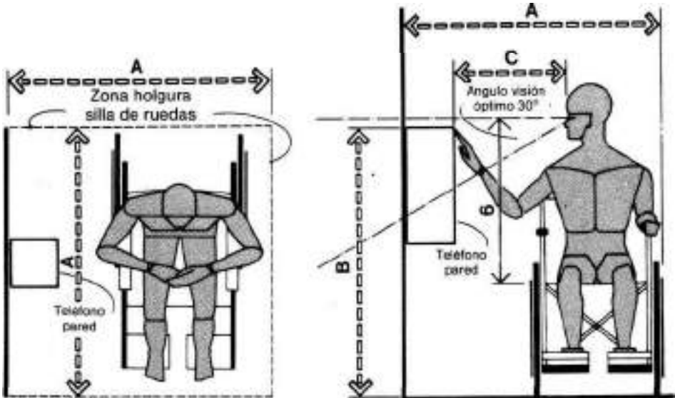
TELÉFONO PÚBLICO /USUARIO DISMINUIDO FÍSICO
