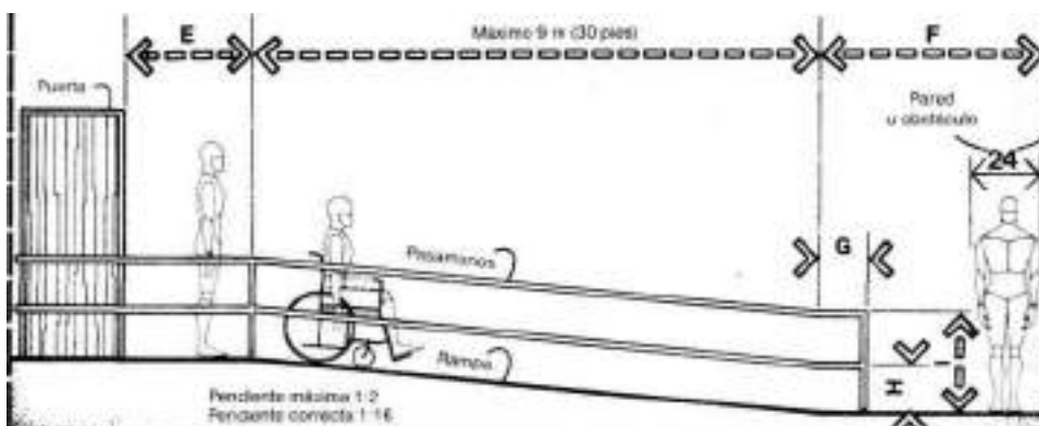
RAMPA DE ACCESO
