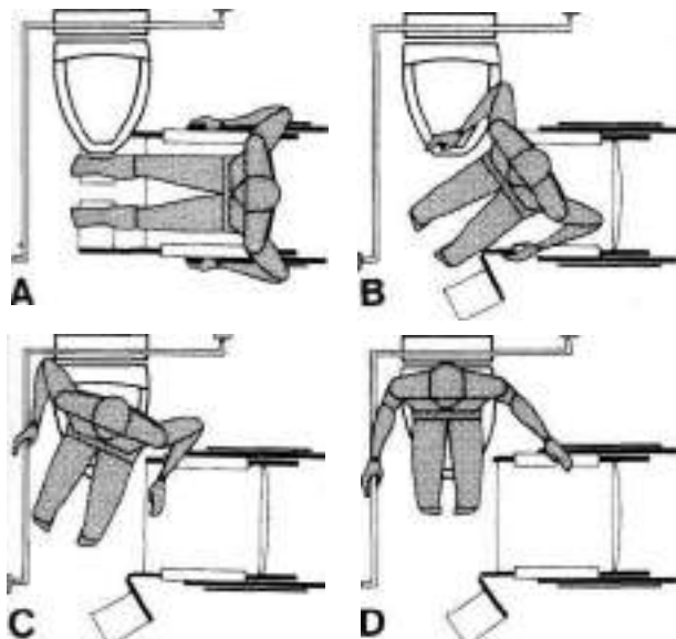
TÉCNICA DE ACCESO CON TRANSFERENCIA LATERAL
