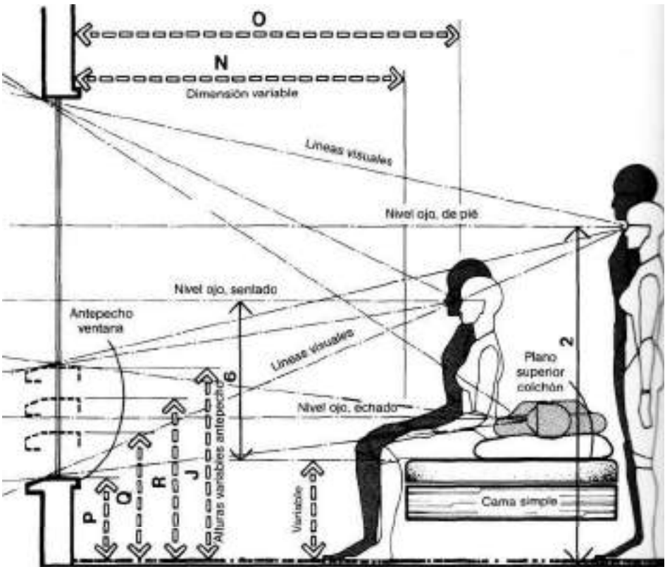
DORMITORIO/VISIÓN Y LÍNEAS VISUALES
