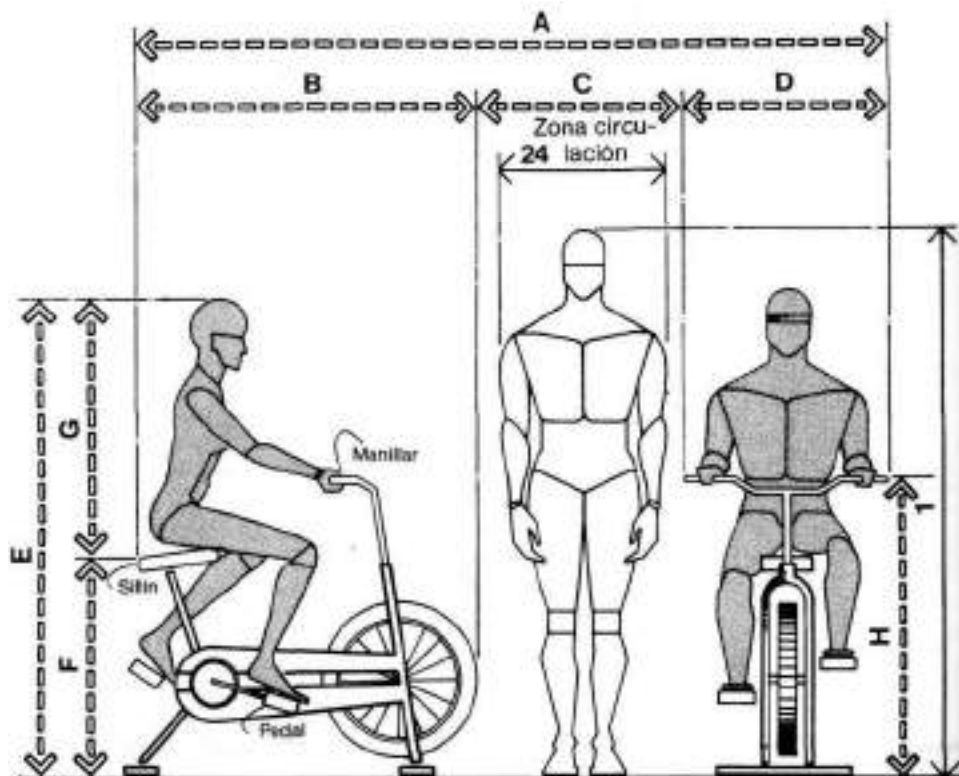
EJERCICIO EN BICICLETA
