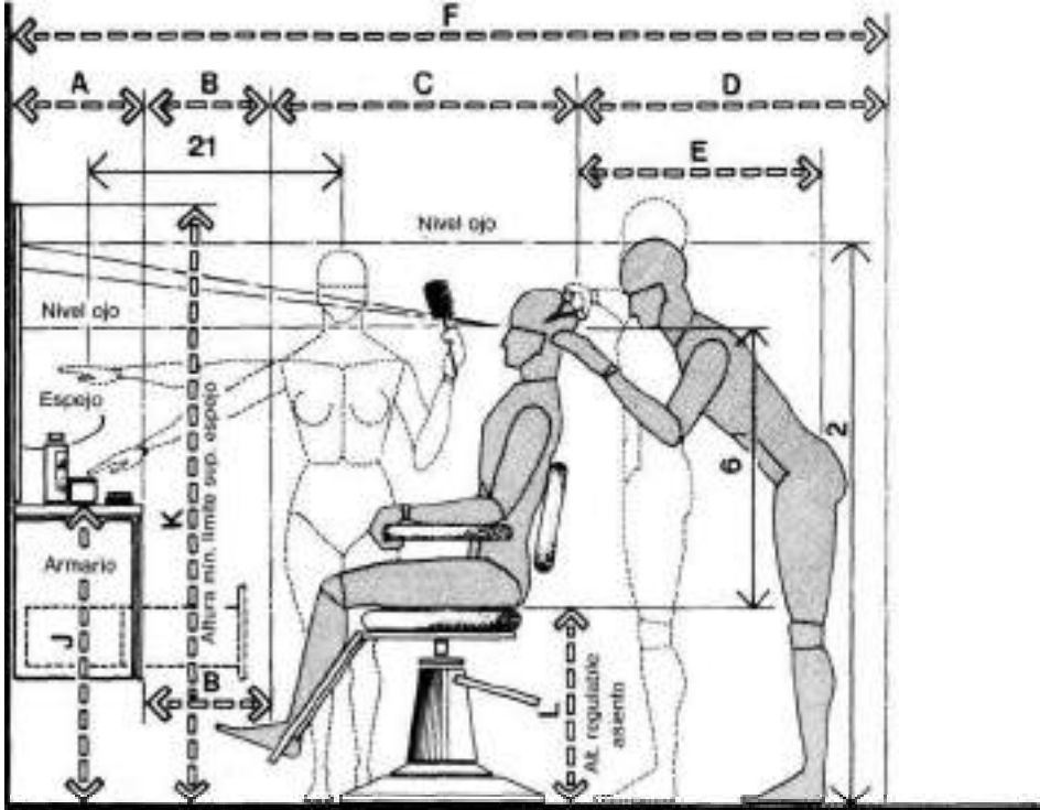
MÓDULO DE TRABAJO EN PELUQUERÍA
