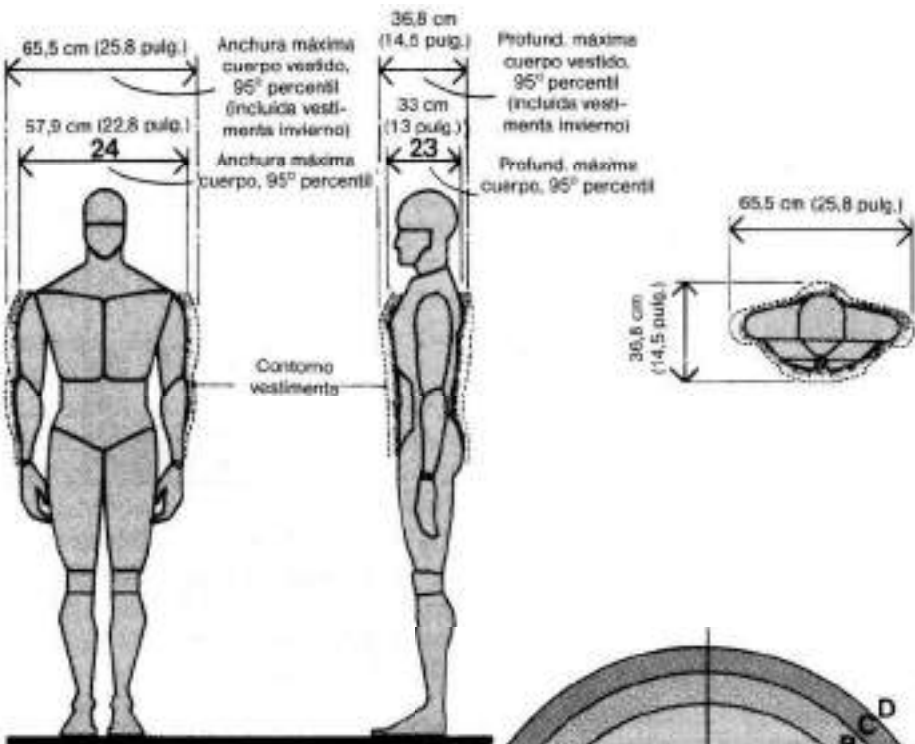
EL CUERPO HUMANO/ PROFUNDIDAD Y ANCHURA
