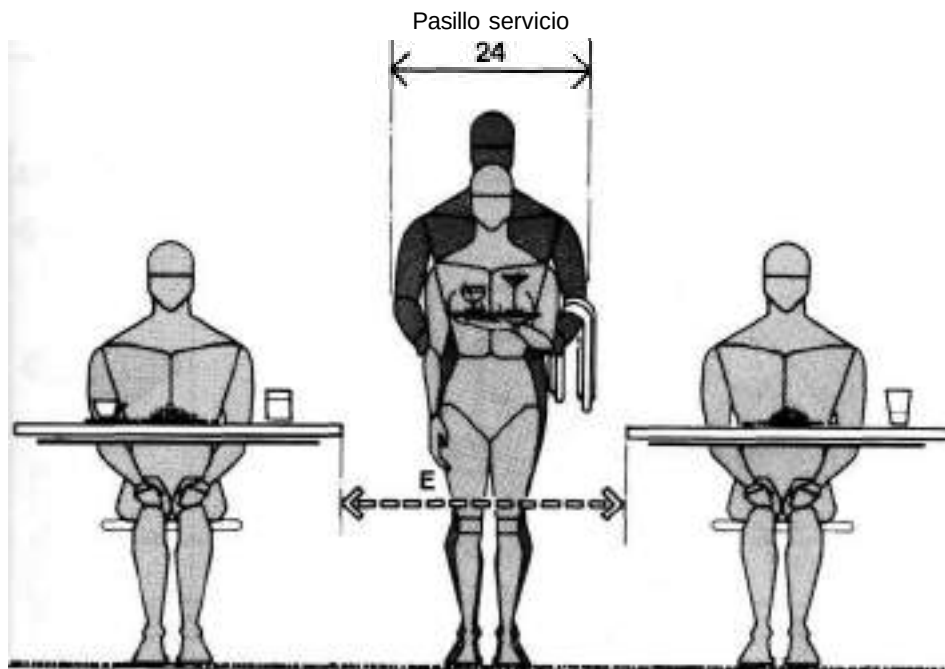
PASILLO DE SERVICIO/HOLGURA ENTRE MESAS
