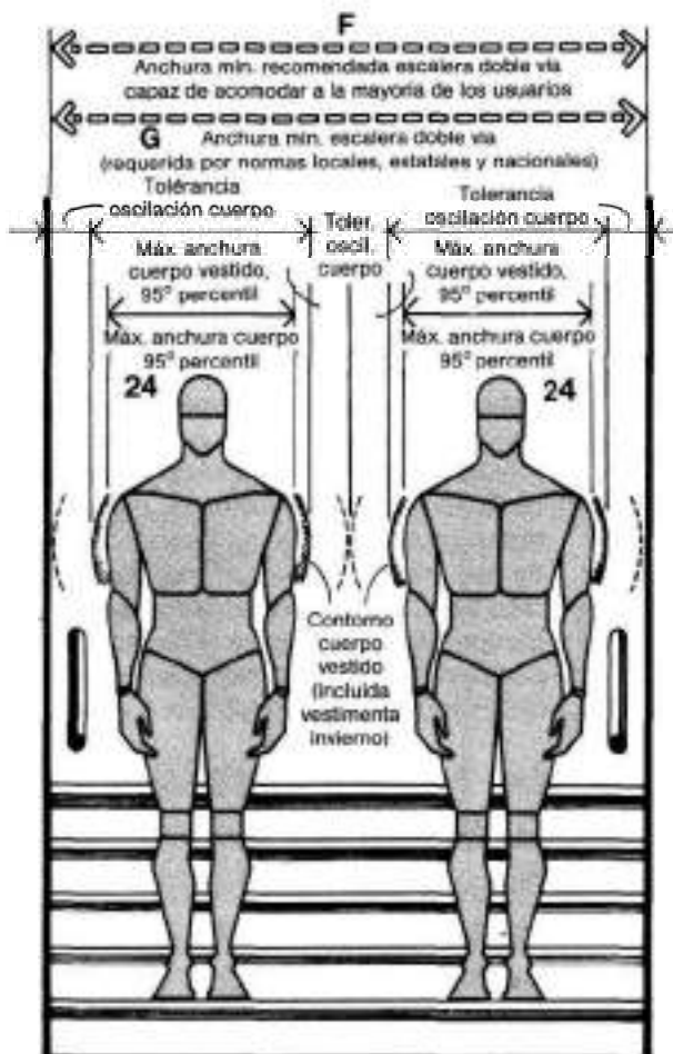
ESCALERAS/ANCHURA EXISTENTE Y RECOMENDADA PARA VÍA DOBLE
