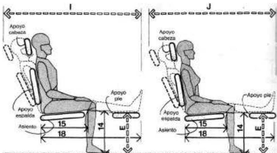
SILLA RECLINABLE CON APOYAPIES/HOMBRE Y MUJER
