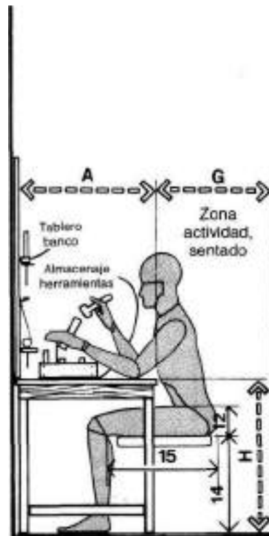
BANCO DE TRABAJO BAJO
