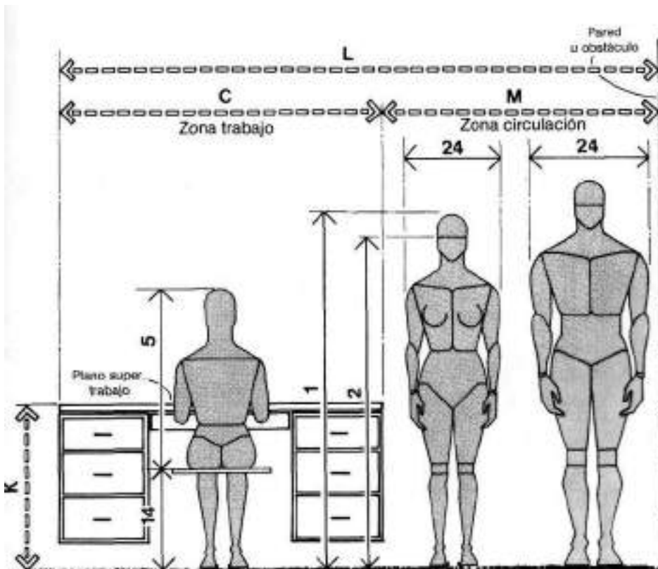
MODULO DE TRABAJO Y CIRCULACIÓN ADYACENTE
