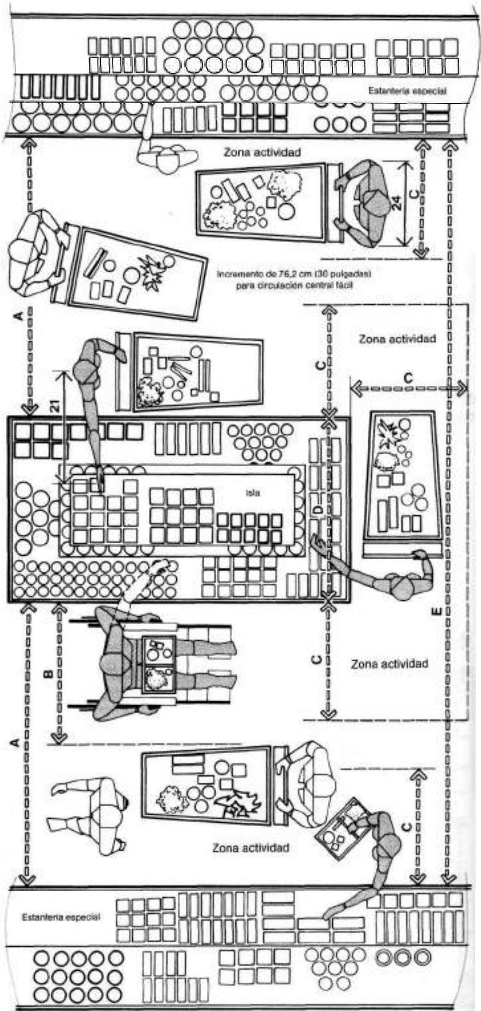
HOLGURAS EN PASILLOS
