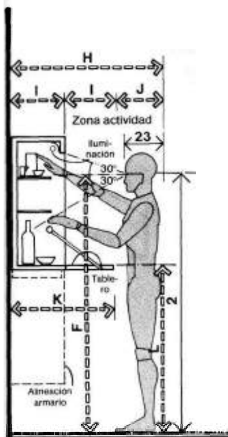
MUEBLE BAR PARED/ ACCESO HOMBRE
