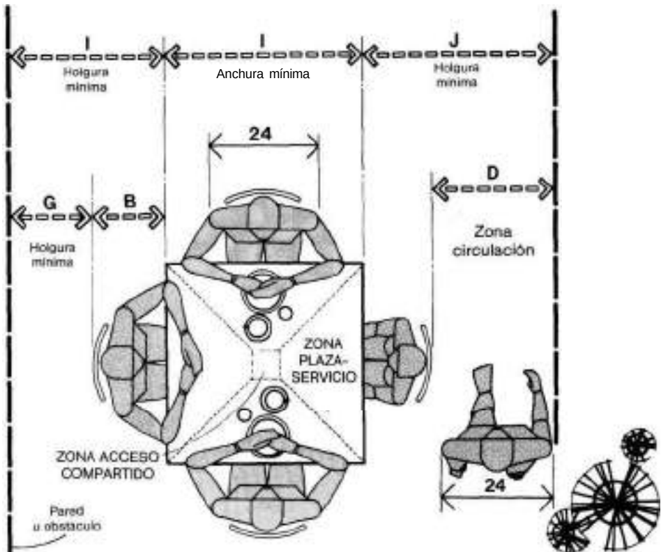
MESA DE DESAYUNO/COCINA PARA CUATRO PERSONAS
