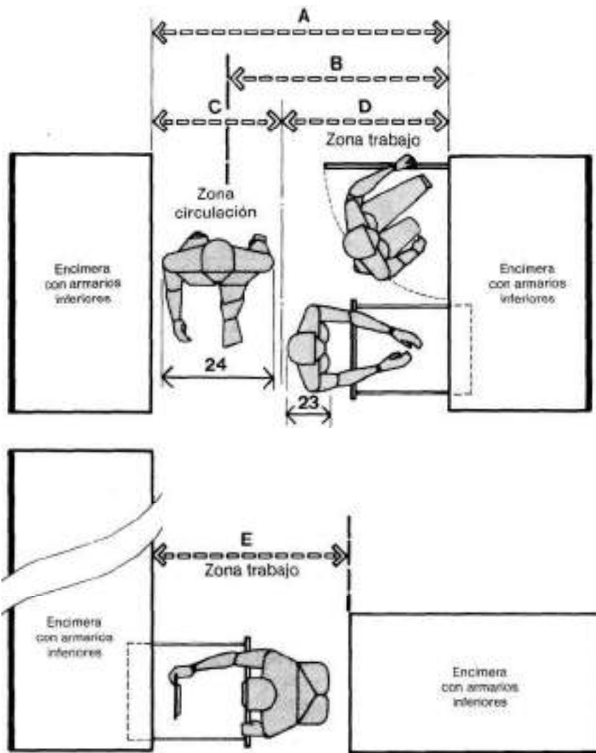
MOBILIARIO DE COCINA/ HOLGURA GENERAL
