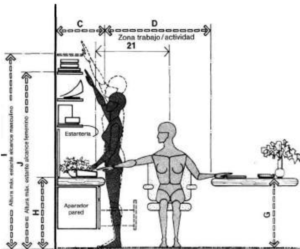
CONSIDERACIONES SOBRE MESA DE DESPACHO/APARADOR
