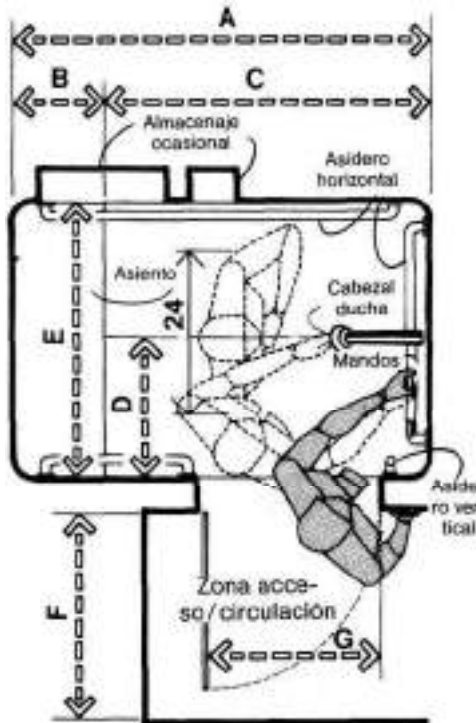
HOLGURAS MÍNIMAS PARA DUCHAS
