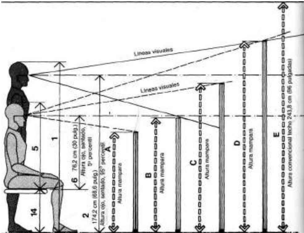
DIVISORIAS VISUALES/CONSIDERACIONES ANTROPOMÉTRICAS MASCULINAS
