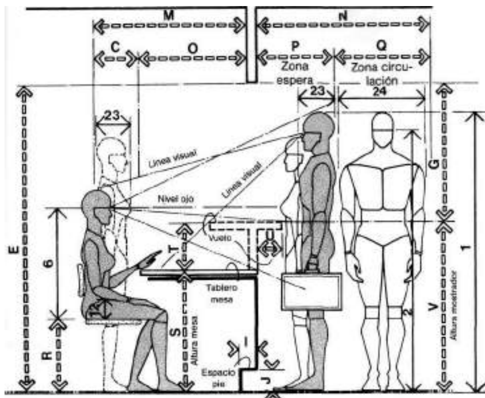
MÓDULO DE RECEPCIÓN/ALTURA DE LA MESA
