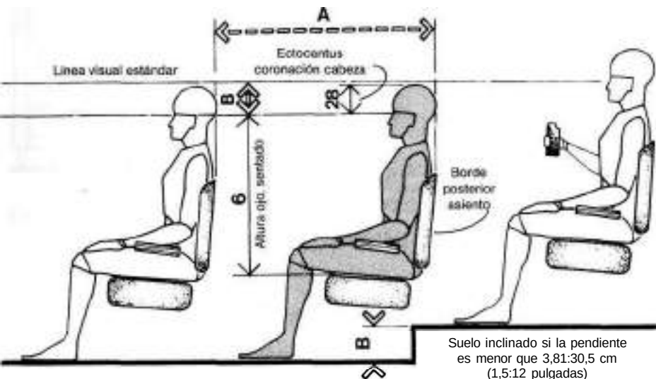
ASIENTO ESCALONADO/VISION DE DOS FILAS
