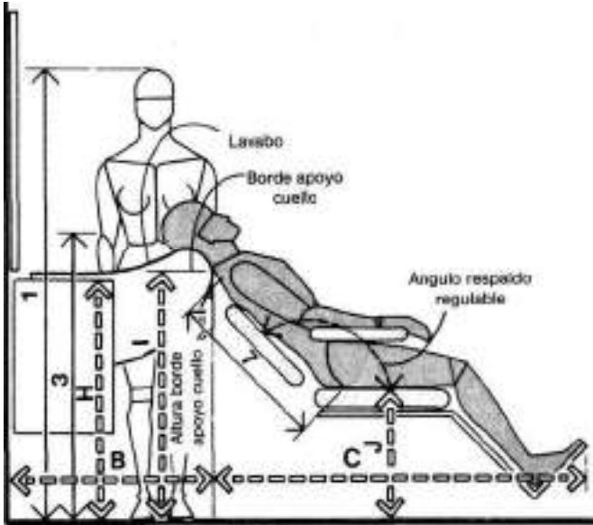
MÓDULO DE LAVADO/CLIENTE MASCULINO
