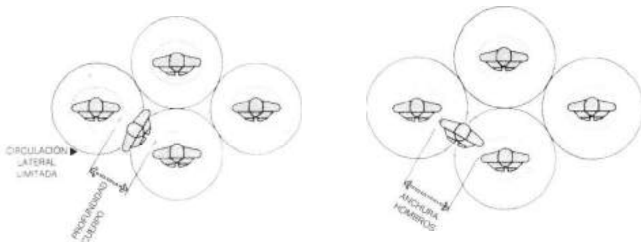
Fig. 2-6 (izquierda). Ilustración de la "zona de confort personal", de Fruin, con aumento de la "zona tope" a 106,7 cm (42 pulgadas) de diámetro y 0,93 \text{ m}^2 (10 pies 2 ) de superficie. Las personas en pie están separadas por toda una profundidad corporal, teniendo en cuenta una circulación lateral reducida por desplazamiento lateral. Fig. 2-7 (derecha). Ilustración de la "zona de circulación", de Fruin, con aumento de la zona tope a 121,9 cm (48 pulgadas) de diámetro y 1,21 \text{ m}^2 (13 pies 2 ) de superficie. Fruin afirma que de 0,93 a 1,21 m (10 a 13 pies) por persona permitiría circular sin molestar a nadie.
