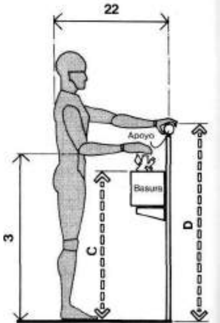
PAPELERA/ USUARIO DISMINUIDO FÍSICO CON MOVILIDAD
