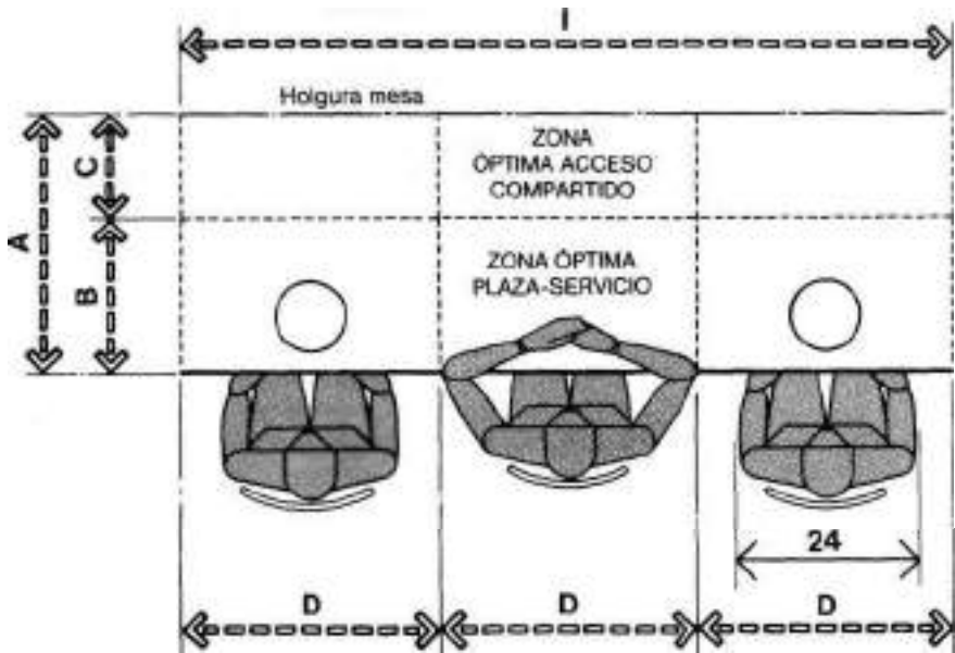
PLAZA DE SERVICIO ÓPTIMA PARA TRES PERSONAS
