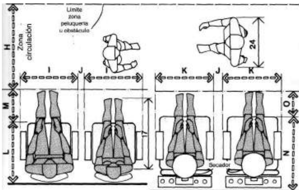
ZONA DE ESPERA Y CIRCULACIÓN/HOLGURAS
