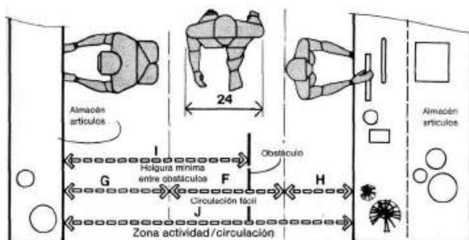
ANCHURAS DE PASILLOS SECUNDARIOS PÚBLICOS
