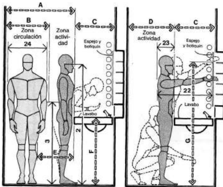
LAVABO/CONSIDERACIONES ANTROPOMÉTRICAS PARA HOMBRE
