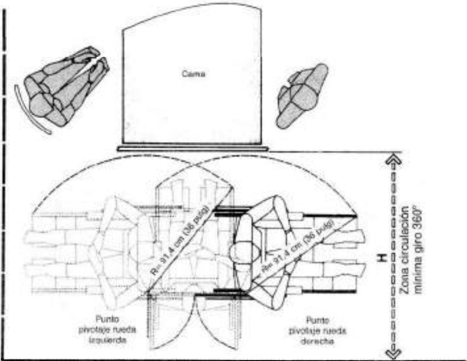
DORMITORIO DE PACIENTE/ESPACIO DE MANIOBRA PARA SILLA DE RUEDAS
