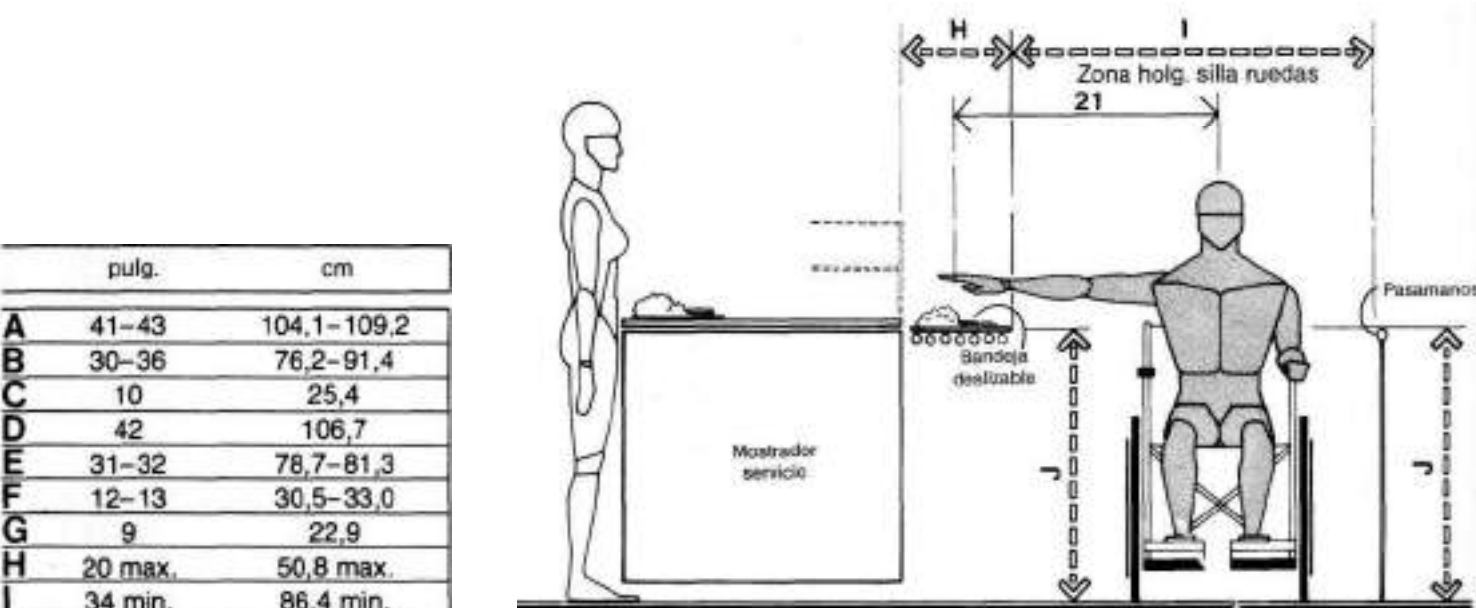
MOSTRADORES AUTOSERVICIO/ACCESO DE SILLAS DE RUEDAS
