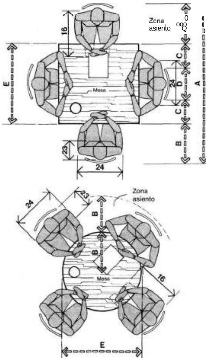
MESAS DE CONFERENCIA/CUADRADA Y CIRCULAR
