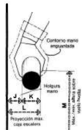
PASAMANOS/DISEÑO RECOMENDADO POR LOS AUTORES
