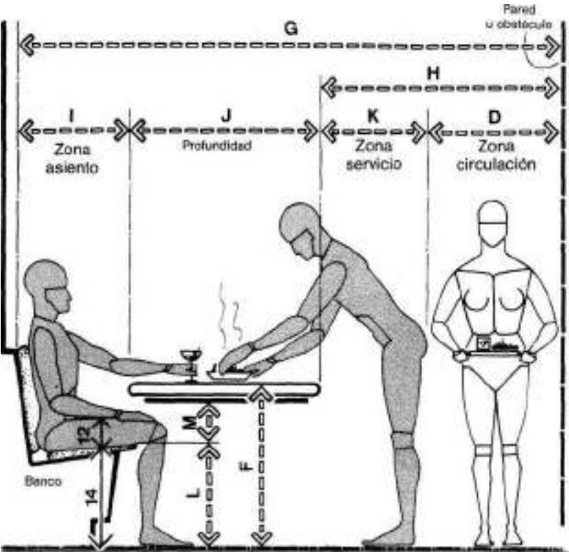
BANCO CORRIDO/HOLGURAS DE SERVICIO Y PASO
