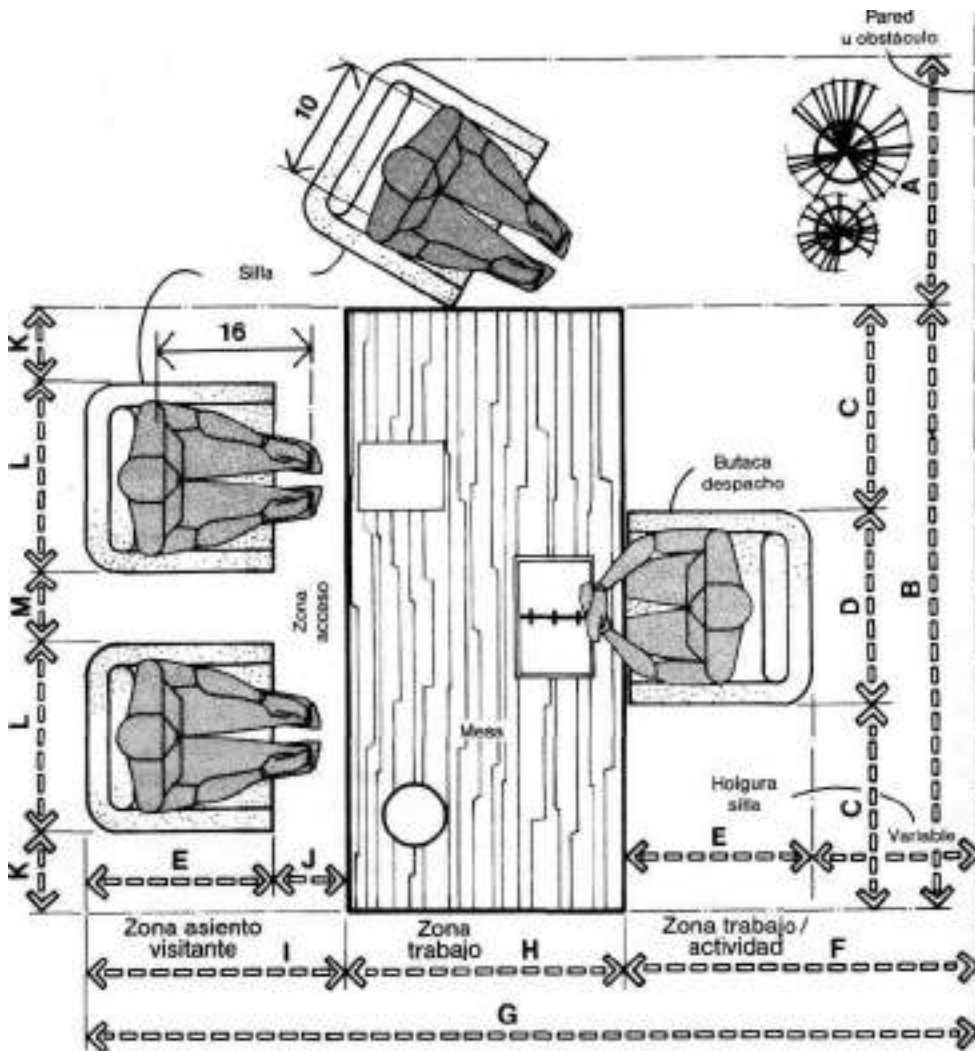
MESA DE DESPACHO/ASIENTO DE VISITANTE
