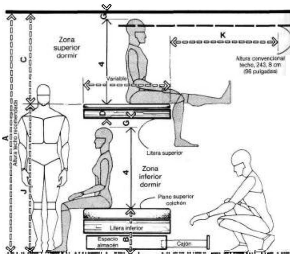
LITERAS PARA ADULTOS/ALZADO LATERAL
