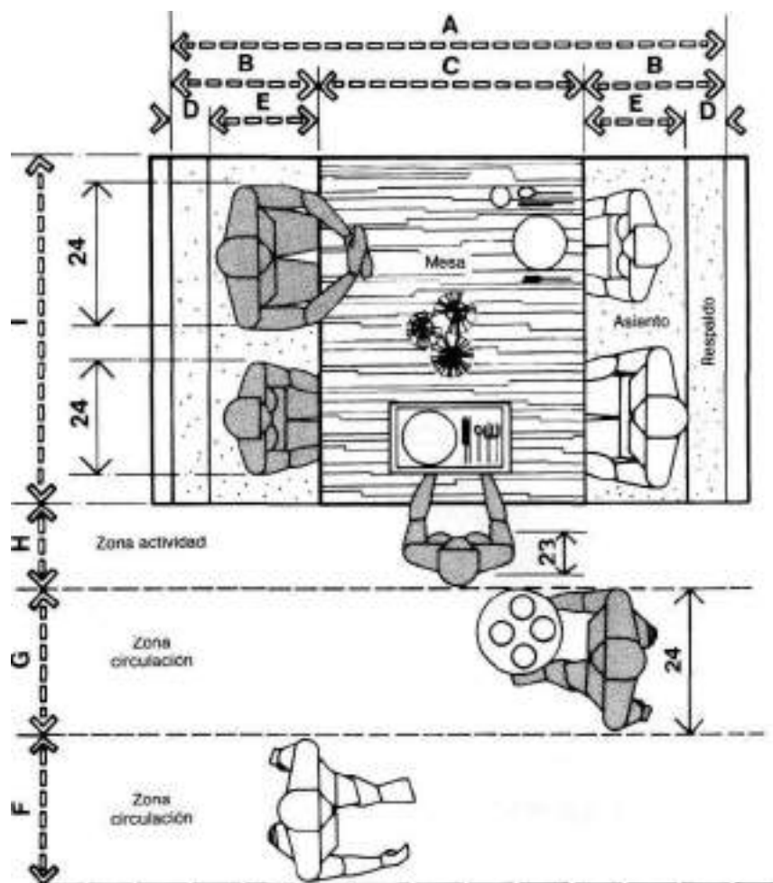
HOLGURAS PARA MÓDULOS DE ASIENTOS Y CIRCULACIÓN
