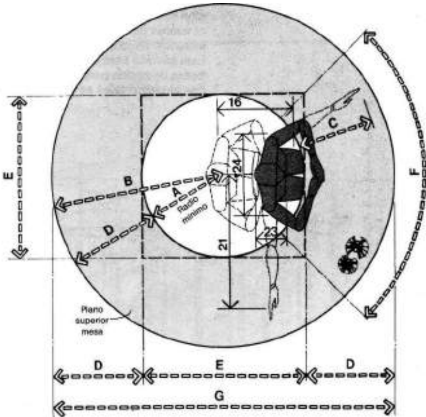
MÓDULO CIRCULAR DE RECEPCIÓN
