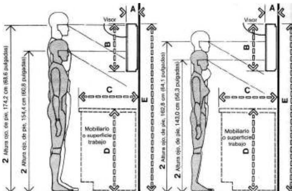
ALTURA DE OJO/OBSERVADORES DE PIE, AMBOS SEXOS, ALTOS Y BAJOS
