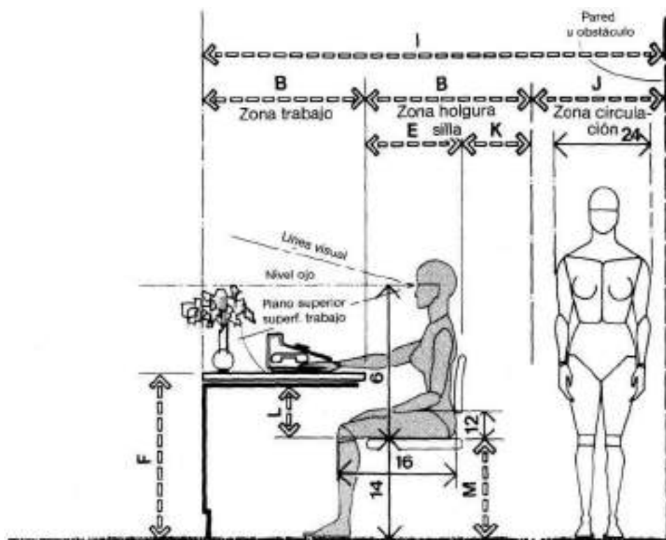
MODULO BÁSICO DE TRABAJO CON CIRCULACIÓN POSTERIOR
