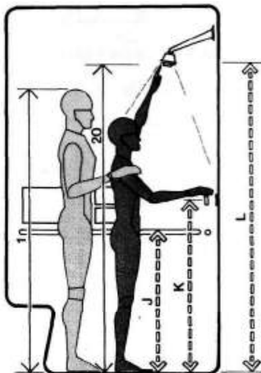
DUCHA/ALCANCE Y HOLGURA
