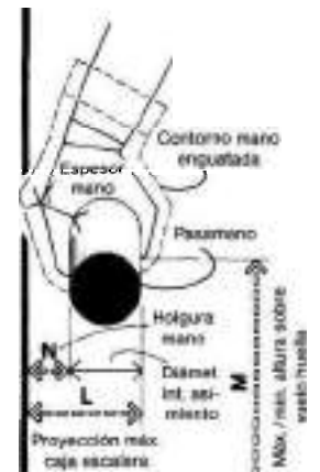
PASAMANOS/ESTUDIO ANTROPOMÉTRICO DE LOS ESTÁNDARES DOMINANTES
