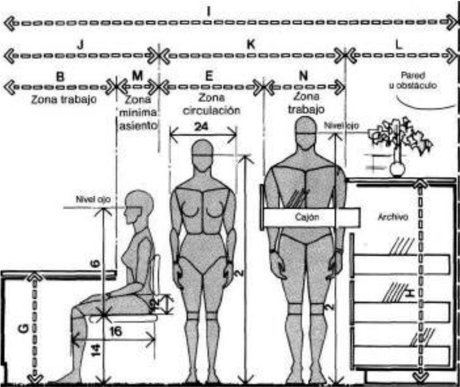
MESA DE DESPACHO CON ARCHIVO Y ALMACENAJE
