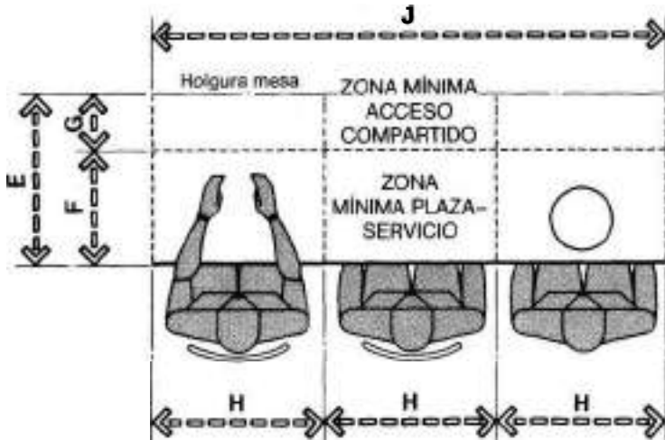
PLAZA DE SERVICIO MÍNIMA PARA TRES PERSONAS
