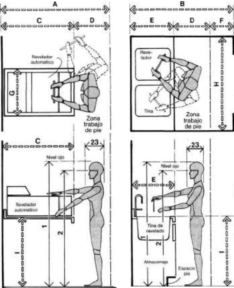
CUARTO OSCURO Y EQUIPO DE REVELADO AUTOMÁTICO
