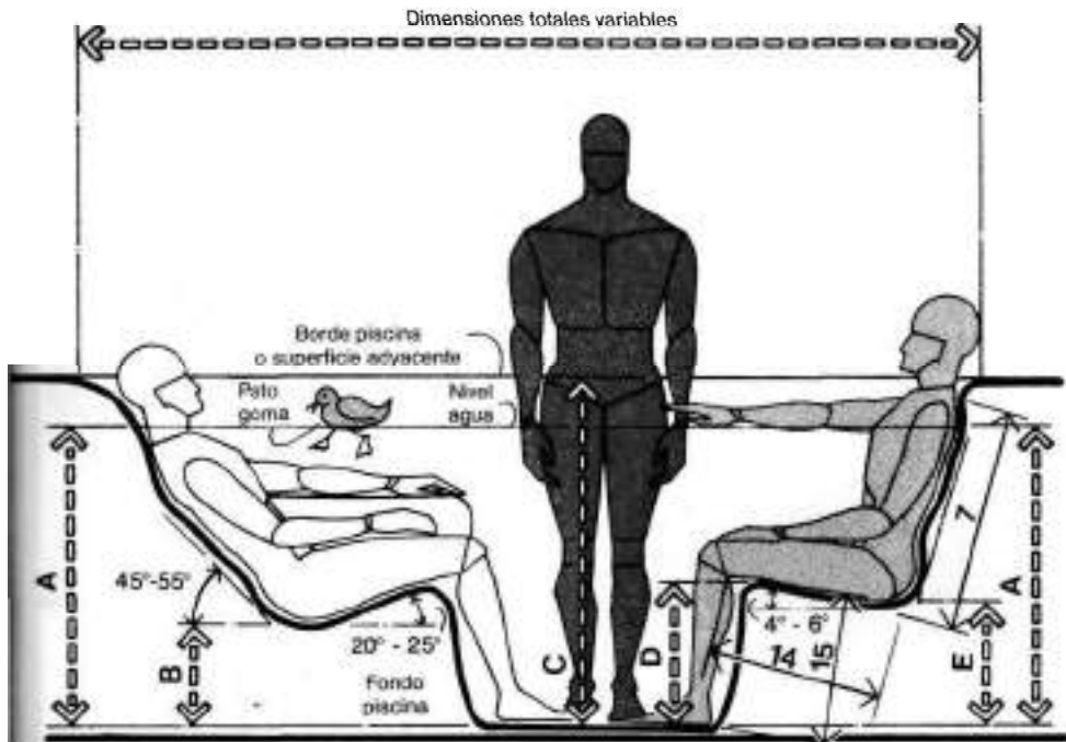
PISCINA PARA HIDROTERAPIA DE DIMENSIONES ANTROPOMÉTRICAS
