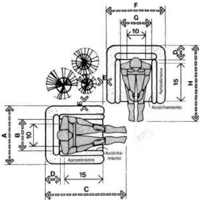
SILLÓN RINCONERA/HOMBRE Y MUJER
