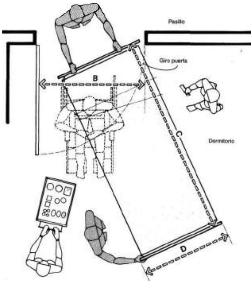
PUERTA DE ACCESO AL DORMITORIO
