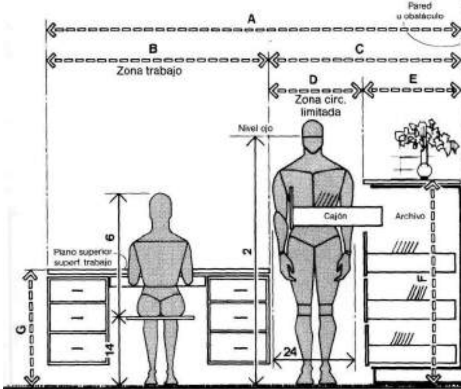
MODULO DE TRABAJO CON ARCHIVO Y ALMACENAJE
