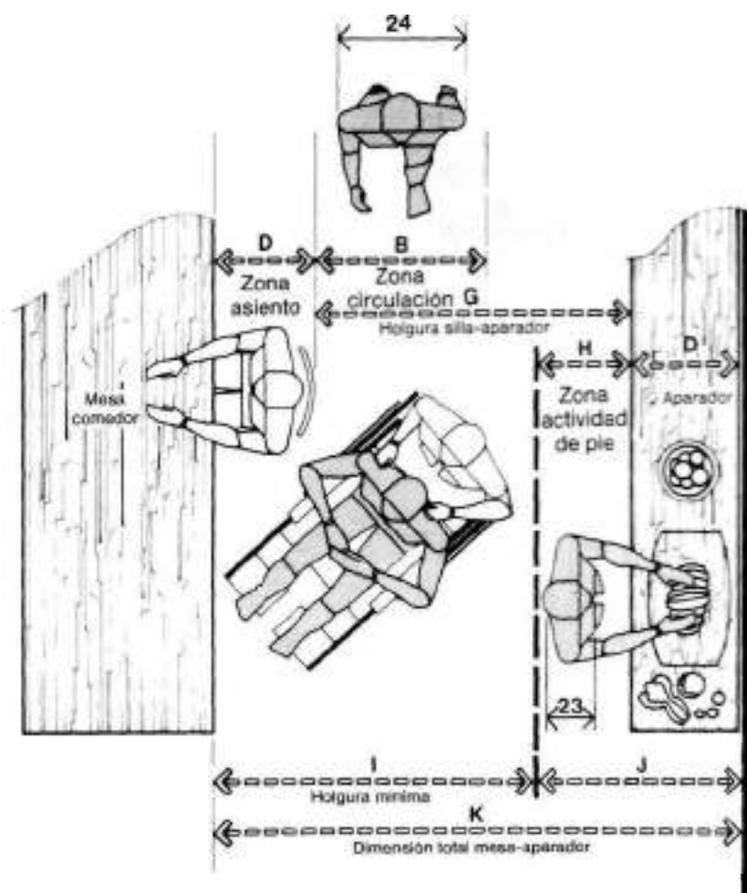
HOLGURAS ENTRE MESA Y APARADOR
