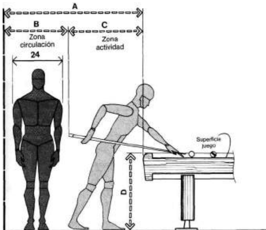
REQUISITOS DE LA MESA DE BILLAR
