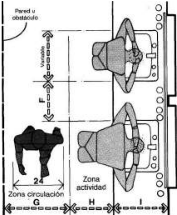
HOLGURAS PARA LAVABO DOBLE
