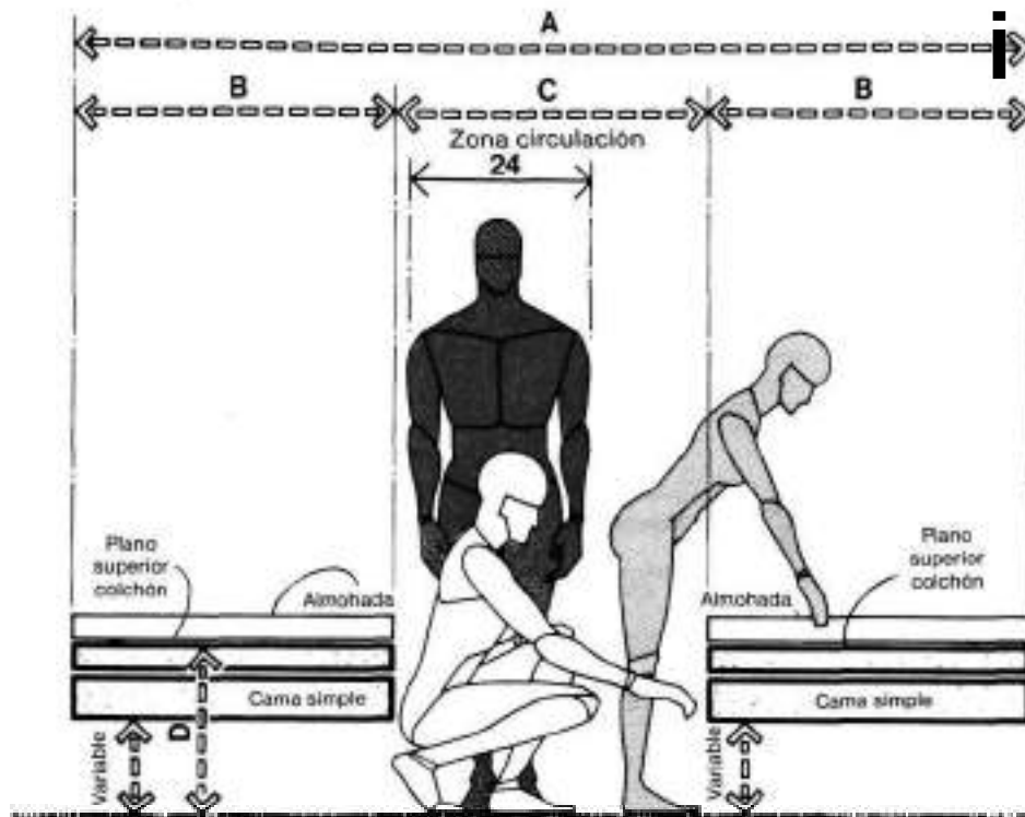
CAMA GEMELA/HOLGURAS Y DIMENSIONES
