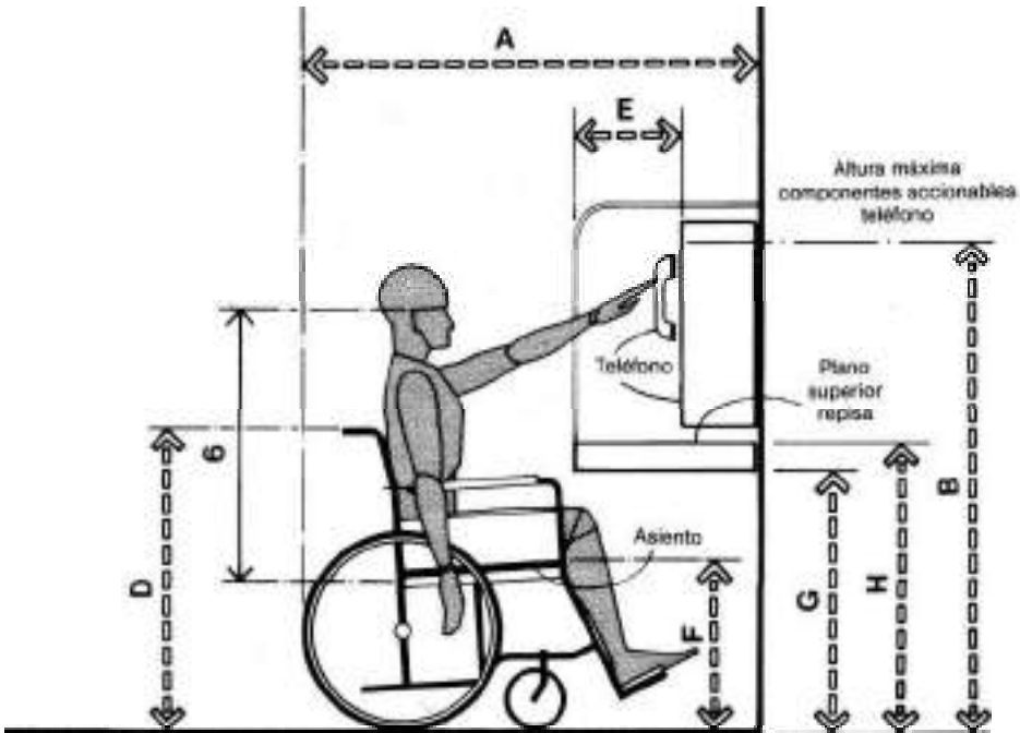
TELÉFONO PÚBLICO /USUARIO DISMINUIDO FÍSICO
