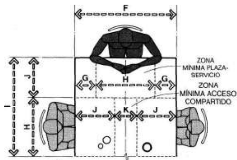
ANCHURA MÍNIMA DE MESA
