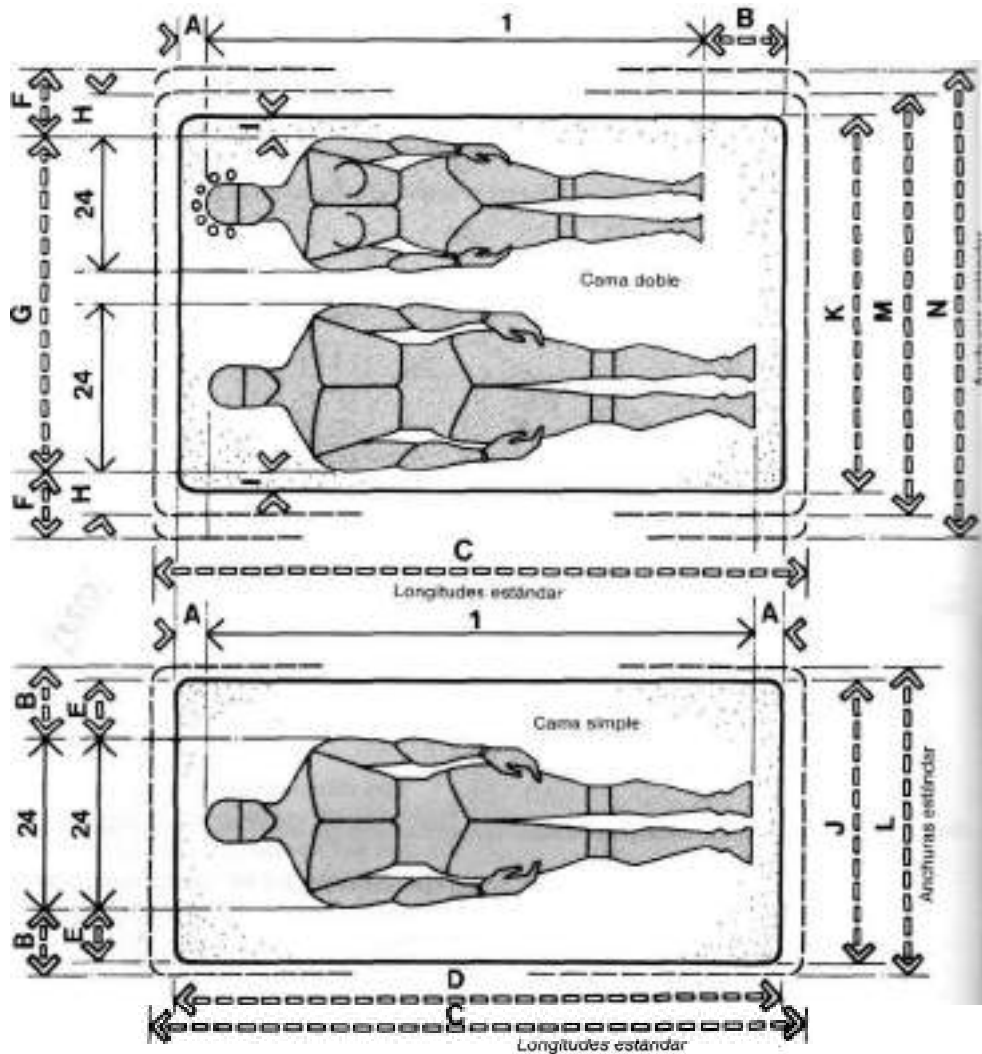
CAMA SIMPLE Y DOBLE
