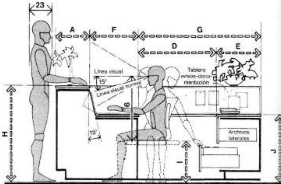
MÓDULO DE ENFERMERAS
