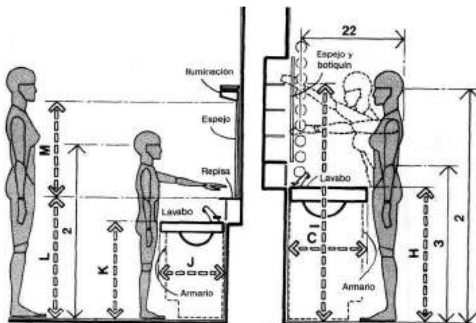
LAVABO / CONSIDERACIONES AMTROPOMETRICAS PARA MUJER Y NIÑOS
