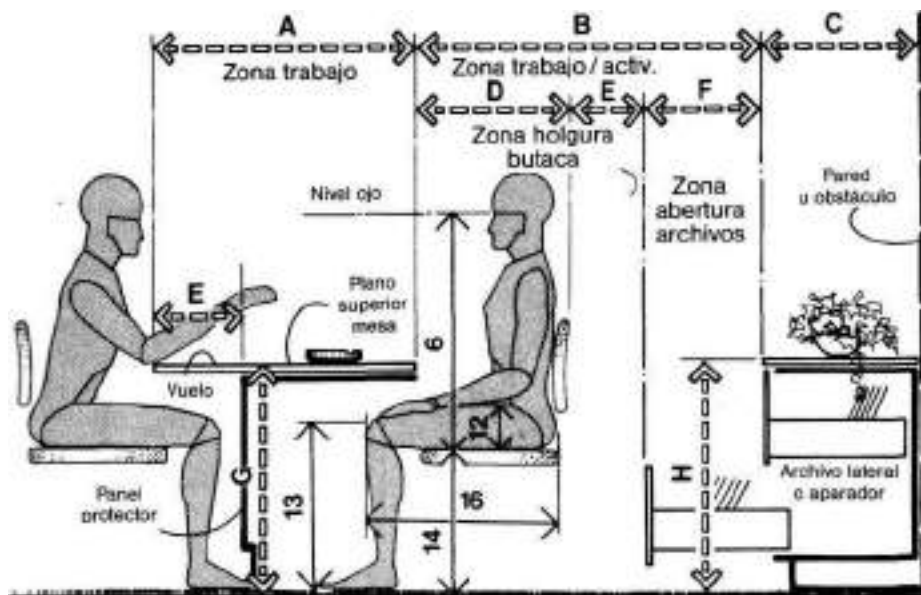
MESA DE DESPACHO/HOLGURAS BÁSICAS
