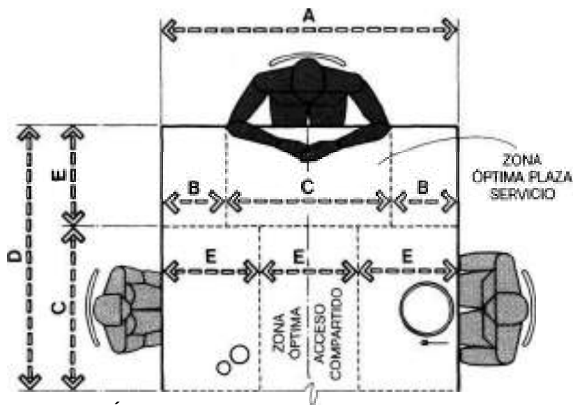
ANCHURA ÓPTIMA DE MESA
