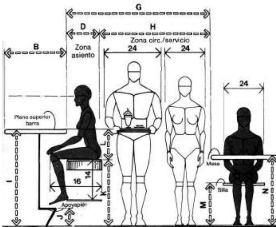
BARRA PARA COMER/HOLGURAS MESAS
