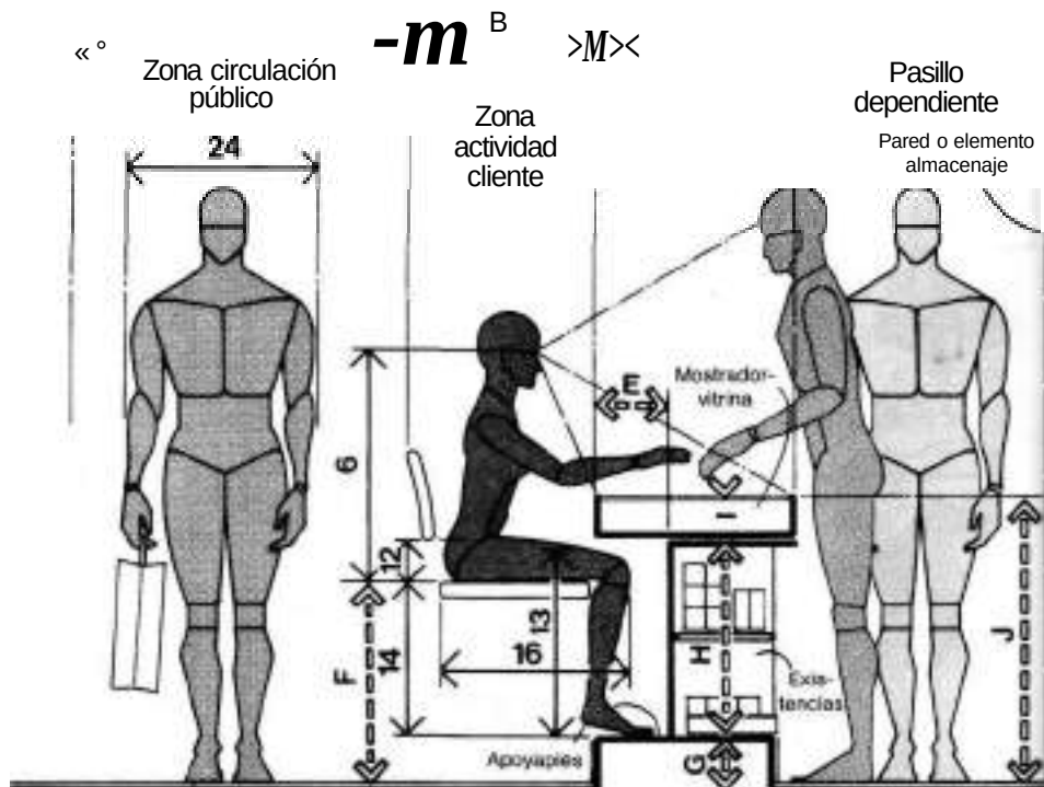
CLIENTE SENTADO/ALTURA DE MOSTRADOR RECOMENDABLE
