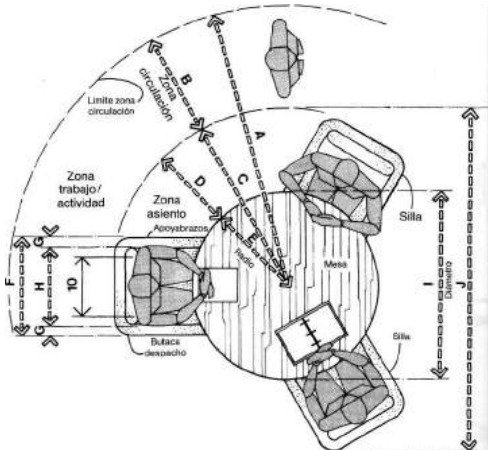
MESA DE DESPACHO CIRCULAR
