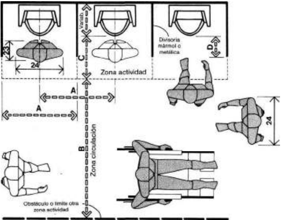
DISTRIBUCIÓN DE URINARIOS
